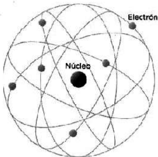
Esquema del modelo de Rutherford (1911).
