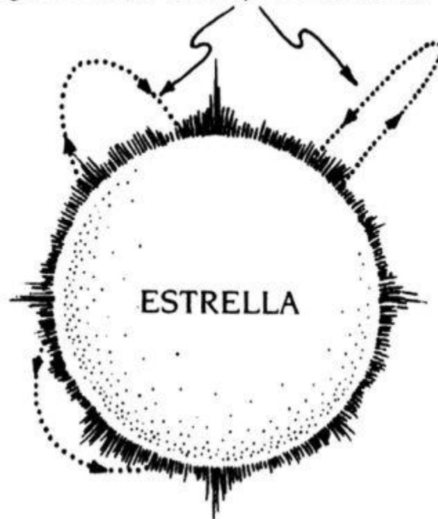
Trayectorias de los corpúsculos de luz
