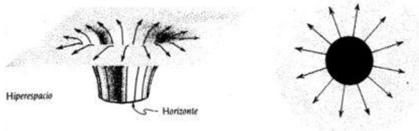
7.6. Líneas de campo eléctrico que emergen del horizonte de un agujero negro eléctricamente cargado. Izquierda: diagrama de inserción. Derecha: vista superior del diagrama de inserción.
