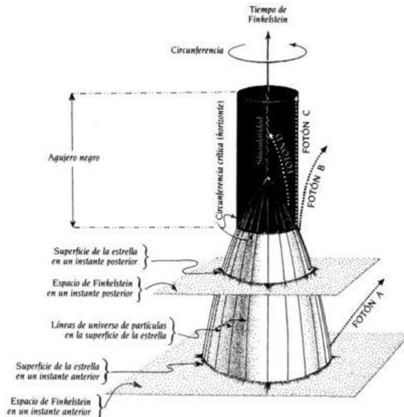
6.7. Un diagrama espacio-temporal que representa la implosión de una estrella para formar un agujero negro. Hacia arriba se representa
