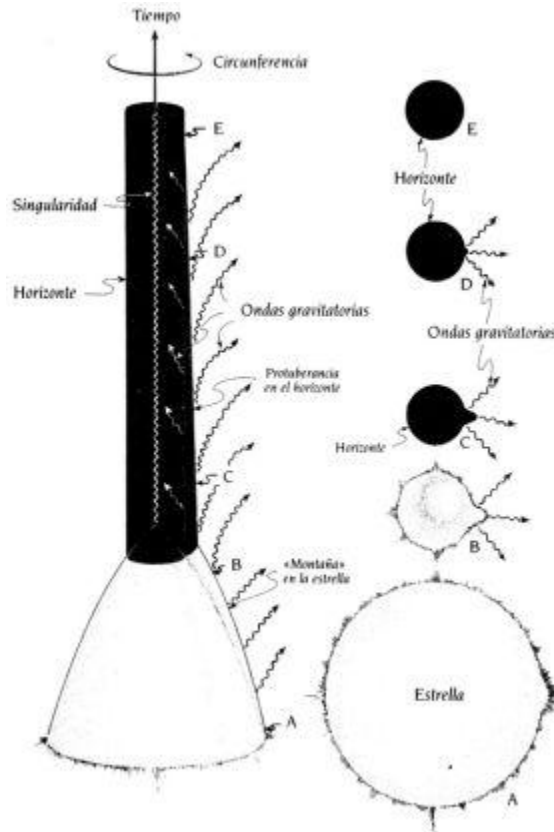
7.4. Diagrama espacio-temporal (izquierda) y una secuencia de instantáneas (derecha) que muestran la implosión de una estrella con una montaña para formar un agujero negro.
