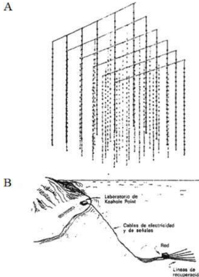
Figura 19. Detector DUMAND de neutrinos procedentes del espacio. A muestra una representación esquemática de una red de foto detectores utilizados para observar los efectos de la interacción submarina de neutrinos con alta energía. B muestra cómo se desplegaría esta red en el océano Pacífico.
