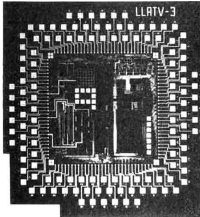
Figura 28. Estructura de micro ingeniería. Chip de computador que contiene conmutadores lógicos y otros circuitos. El chip tiene una longitud total de 4 milímetros, y algunos de los canales a través de los cuales fluyen los electrones tienen una longitud de una micra
