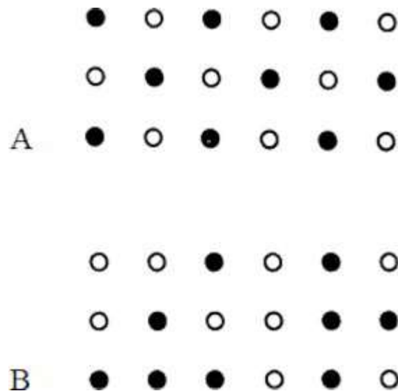
Figura 8. Disposiciones regulares e irregulares. En A aparecen en una estructura regular dos tipos de objetos, representados por círculos blancos y negros. En B aparecen los mismos objetos, en una de las múltiples estructuras irregulares que son posibles.
