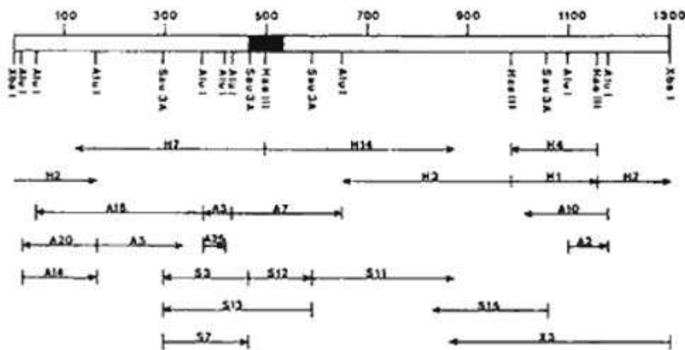
Figura 25. Método para secuenciar el ADN. La barra larga que aparece en la parte superior representa toda la secuencia que se mostraba en la figura 24. Las barras cortas que hay más abajo indican subsecuencias que fueron colocadas juntas mediante un examen de sus regiones de solapamiento.
