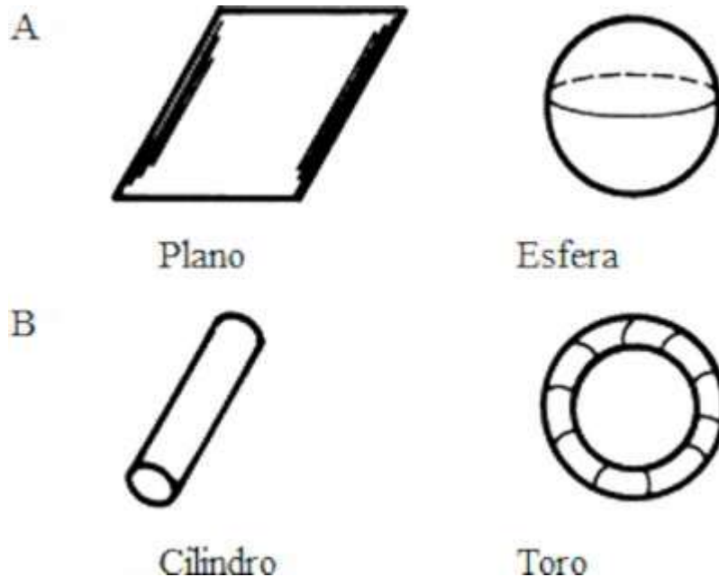
Figura 7. Dos tipos de espacios multidimensionales. Cada espacio consiste en la superficie de la figura que se representa. En A, cada espacio posee dos dimensiones semejantes. En B, los espacios poseen dos dimensiones no semejantes.
