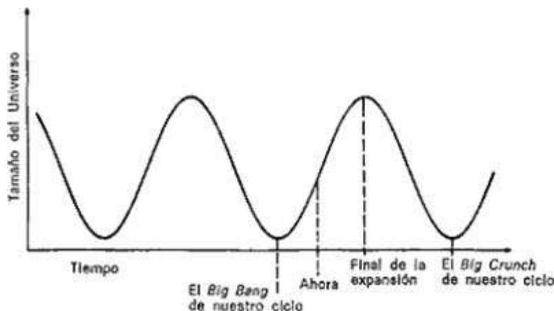
Figura 9. Un Universo oscilatorio. Ésta sería la relación existente entre el tamaño de un Universo y el tiempo, en el caso de un Universo cuyo tamaño aumente y disminuya con periodicidad.
