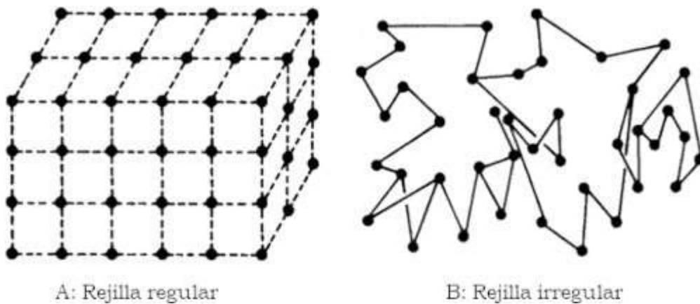
Figura 6. Dos tipos de rejillas tridimensionales. En la rejilla regular A, los puntos están ordenados y conectados de una forma sencilla. En la rejilla irregular B, el orden y las conexiones existentes entre los puntos no se ajustan a un patrón sencillo.
