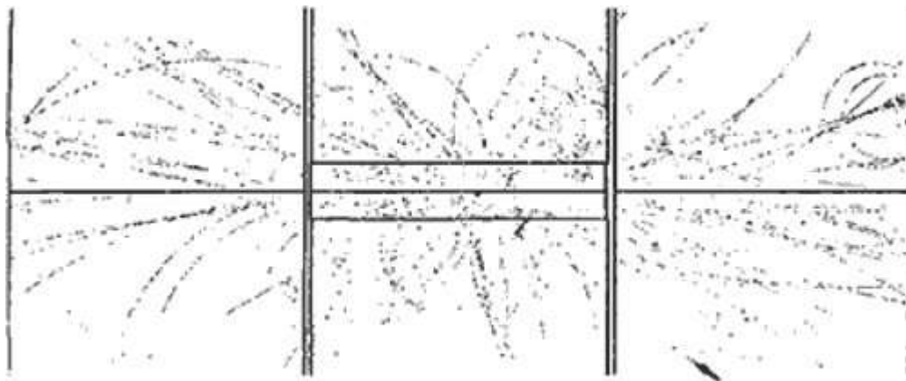
Figura 23. Un acontecimiento complejo en el que intervienen partículas. La fotografía muestra muchos recorridos de partículas que están pasando a través de un detector. Los recorridos han sido reconstruidos mediante un análisis por computador de la salida del detector. Uno de los recorridos, indicado por la flecha, es el camino seguido por un producto de desecho de una partícula subatómica acabada de descubrir.
