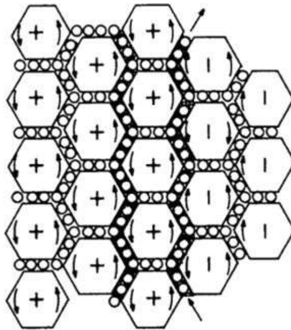
Figura 31. Modelo electromagnético de Maxwell. Los hexágonos representan remolinos, y los pequeños círculos que los rodean son las partículas cargadas de electricidad. Se supone que las partículas y los remolinos giran concéntricamente y producen así el fenómeno que llamamos electromagnetismo.
