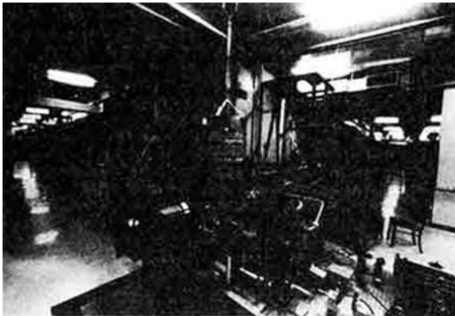
Figura 18. Detector de ondas gravitatorias. En este prototipo de detector de ondas gravitatorias que emplea la interferometría por láser, los haces de láser pasan una y otra vez a lo largo de los largos tubos que aparecen en la imagen, y son analizados por los detectores situados en la jaula de alambre.
