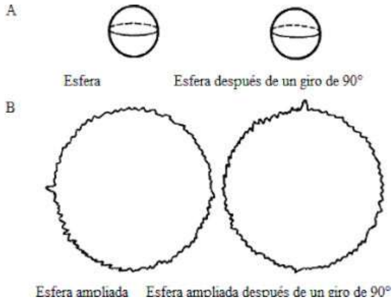
Figura 11. La simetría de una esfera. En A se representa una esfera, junto con la misma esfera después de un giro de 90 grados. A través de una observación a esta escala, no se puede ver ninguna diferencia, y se dice que la esfera permanece invariada después de la rotación. En B se representa con gran aumento la misma esfera, antes y después del giro. Puede apreciarse que a esta escala la simetría de rotación ya no es perfecta, puesto que cambian de posición muchos rasgos de la superficie.
