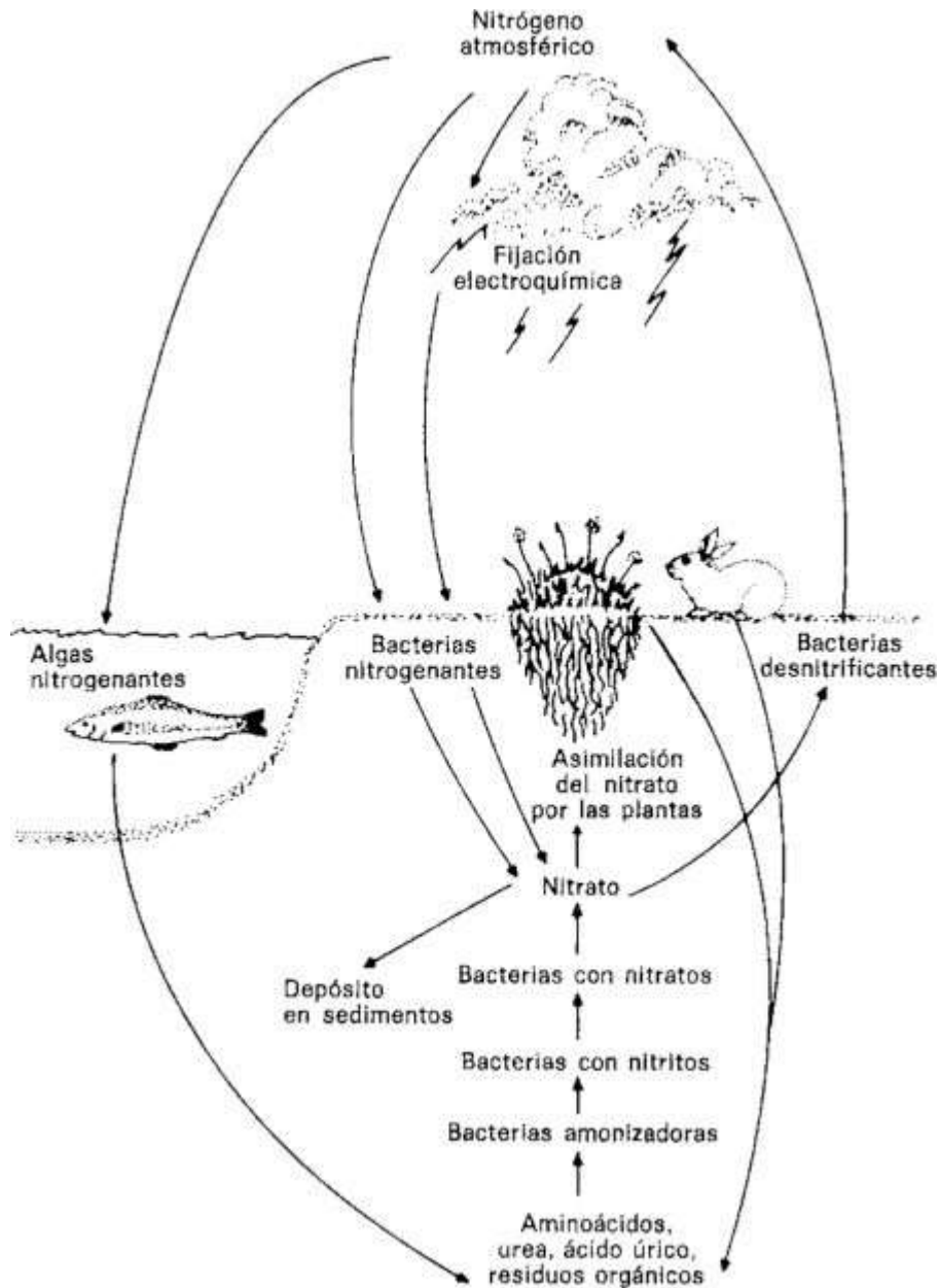
Figura 4. El ciclo del nitrógeno en la biosfera. La figura muestra algunas de las formas en que el nitrógeno fluye desde la atmósfera a través del suelo y de los seres vivos, y vuelve más tarde a la atmósfera.
