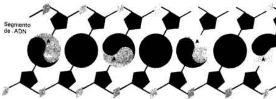
Figura 3. Un modelo de ADN. La cadena de fosfatos y de azúcares de cada lado se sitúa en el exterior, mientras que las bases —A, C, G y T— se sitúan en el interior, unidas a las dos cadenas externas de acuerdo con la regla A-T, G-C.
