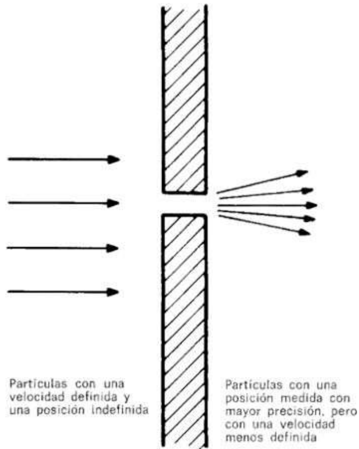
Figura 2. Principio de incertidumbre de Heisenberg. Un dispositivo de medida, por ejemplo, el pequeño orificio practicado en la pantalla, que nos brinda un mayor conocimiento con respecto a la posición de las partículas de un haz, provoca una disminución del conocimiento acerca de las velocidades de estas mismas partículas, debido a la interacción entre dicho dispositivo y las partículas.
