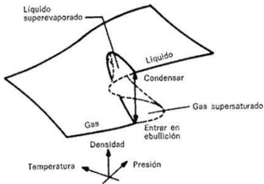
Figura 22. Uno de los tipos de catástrofes. La densidad de una sustancia puede variar de manera continuada a medida que su temperatura cambia, siguiendo la superficie lisa. Para ciertas gamas de temperaturas, pueden existir dos valores de la densidad, y la sustancia puede pasar bruscamente de un valor a otro (en el fenómeno de la ebullición o la condensación), tal como indica la flecha de dos puntas.
