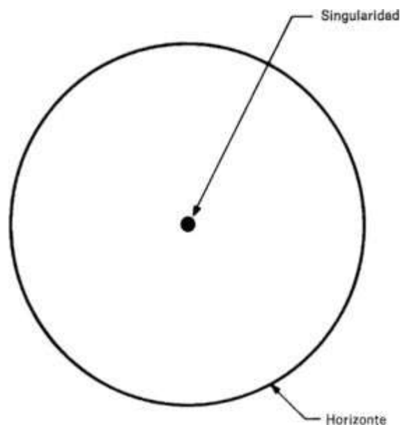
Figura 5. Un agujero negro simple. El horizonte es una esfera imaginaria a través de la cual sólo se efectúan viajes en una dirección. En la región próxima al centro de la esfera, llamada su singularidad, todavía no sabemos qué es lo que sucede.
