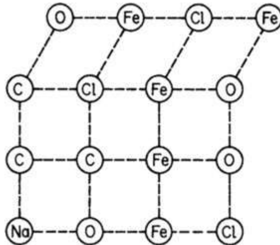
Figura 27. Diagrama parcial de una estructura hipotética de nanoingeniería. El diagrama indica qué átomo hay que colocar en los diversos lugares de una rejilla cúbica.
