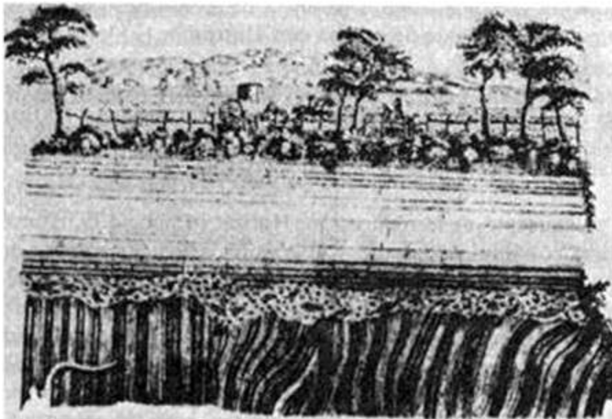
5. Ilustración original de Hutton de una discordancia angular.
