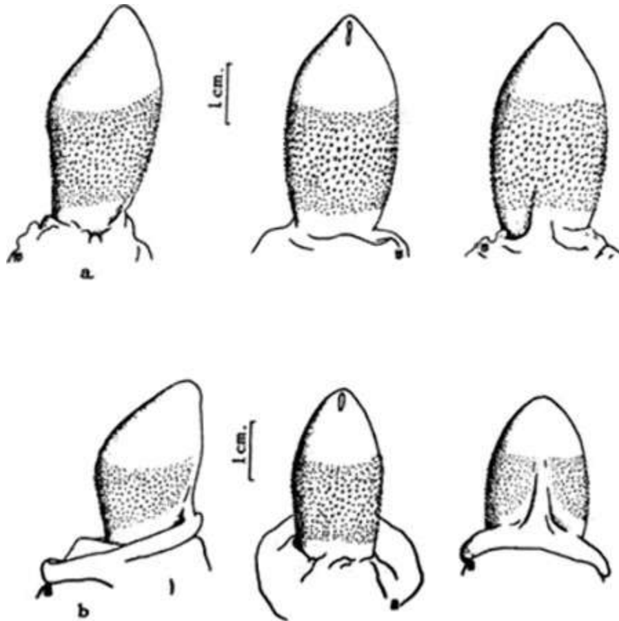
10. Similitud entre los genitales del macho y de la hembra en la hiena manchada. Hilera superior, aspectos del pene del macho. Hilera inferior, aspectos similares del clítoris de la hembra (de Harrison Matthews, 1939).
