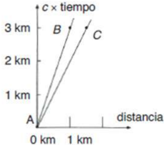
Figura 6. Diagrama espaciotemporal para el sistema de referencia de la granjera.
