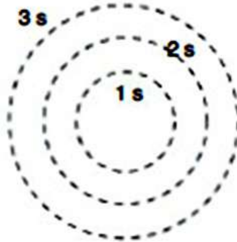
Figura 15. Un horizonte esférico en expansión en el espacio-tiempo de Minkowski.
