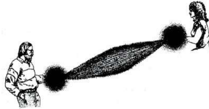
Figura 25. La autodestrucción de una máquina del tiempo en el momento en que es activada por primera vez. [Dibujo de Matthew Zimet en Agujeros negros y tiempo curvo, de Kip Thorne, reproducido con autorización].
