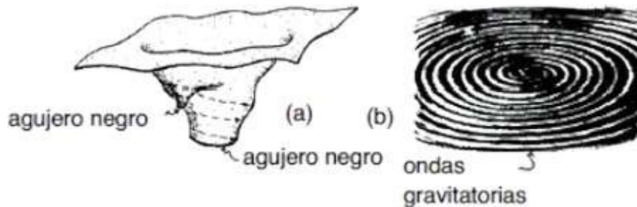
Figura 4. (a) Un agujero negro pequeño en órbita en torno a un agujero negro grande. (b) Las ondas gravitatorias producidas por el movimiento orbital del agujero negro pequeño.
