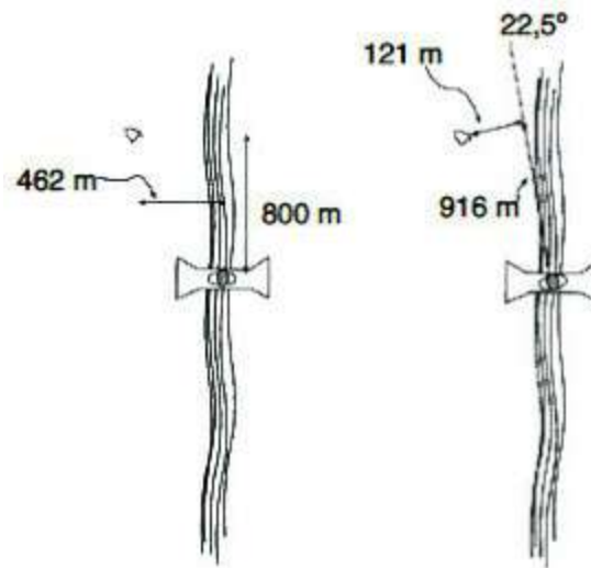
Figura 1. La misma localización con diferentes coordenadas.
