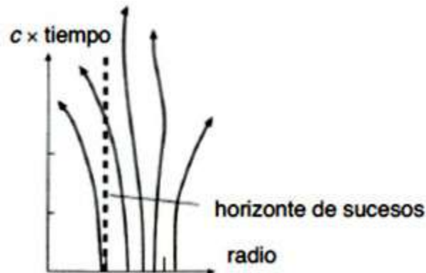
Figura 16. Un horizonte de sucesos de Schwarzschild.
