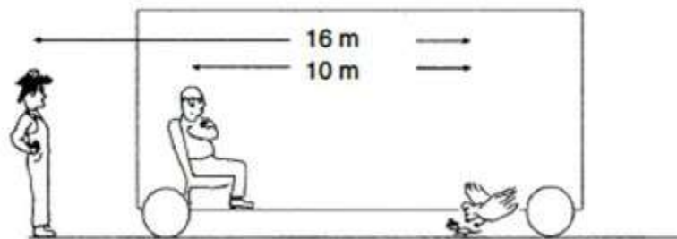
Figura 3. Un suceso observado en dos sistemas de referencia diferentes.
