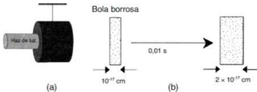
Figura 17. Las consecuencias del principio de incertidumbre para medidas sucesivas del centro de masas de un espejo LIGO avanzado.
