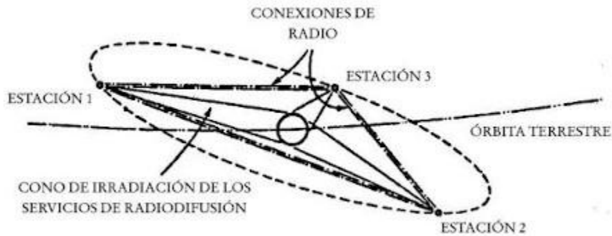
Figura 3. Tres estaciones satélite asegurarán la cobertura completa del globo.
