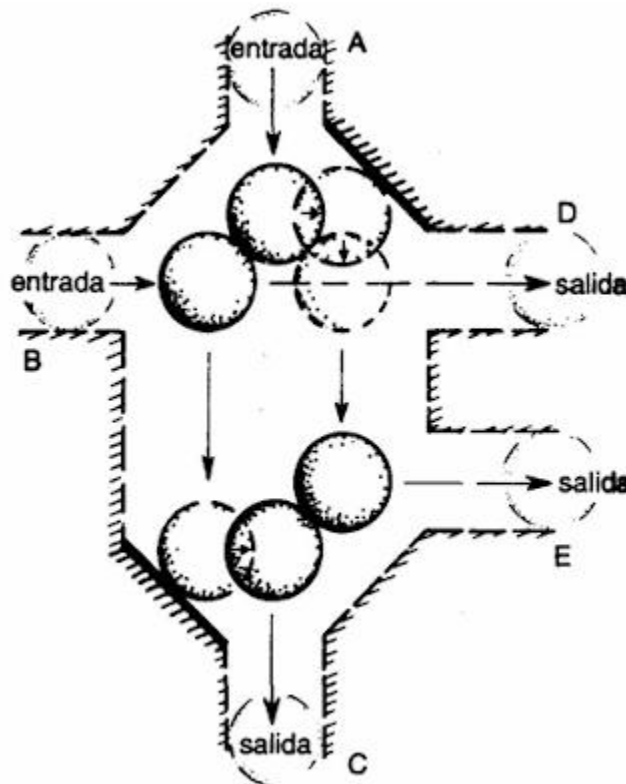
Figura V.9. Un conmutador (sugerido por A. Resler) en la computadora de bolas de billar de Fredkin-Toffoli. Si una bola entra por B, otra saldrá a continuación por D o por E dependiendo de si otra
