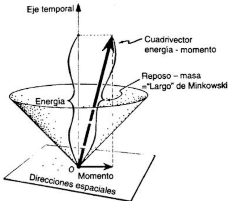
Figura V.35. El cuadrivector energía-momento.
