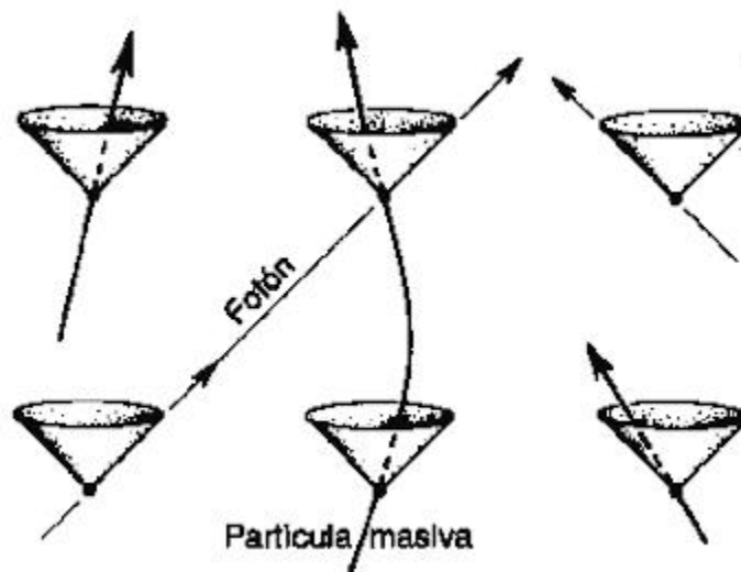
Figura V.17. Imagen de la geometría minkowskiana
