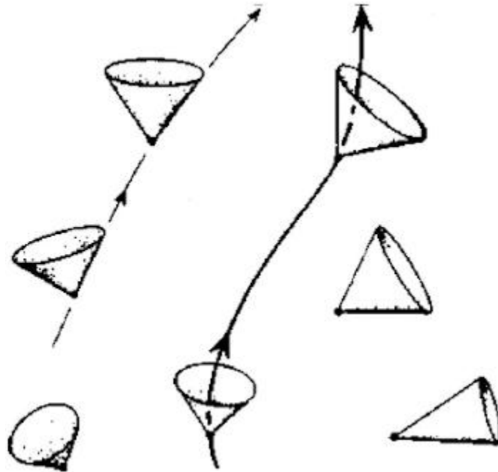
Figura V.29. Representación del espacio-tiempo curvo.
