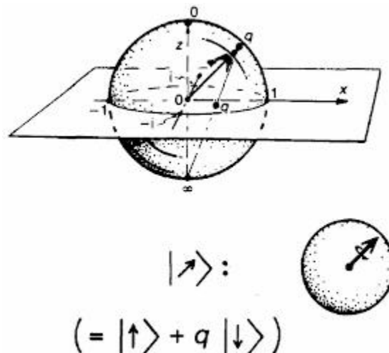
Figura VI.25. La esfera de Riemann, representada aquí como el espacio de estados físicamente distintos de una partícula de spin 1/2 . La esfera se proyecta estereográficamente desde su Polo Sur () en el plano de Argand que pasa por su ecuador.
