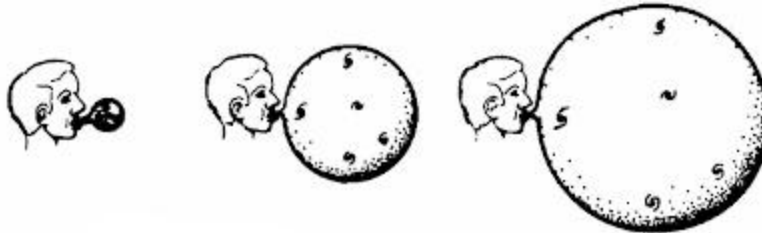
Figura VII.8. Se puede hacer una analogía entre la expansión del Universo y la superficie de un globo que se hincha. Todas las galaxias se alejan una de otra.
