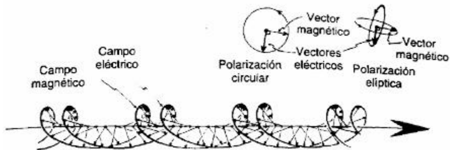
Figura VI.27. Una onda electromagnética circularmente polarizada.
