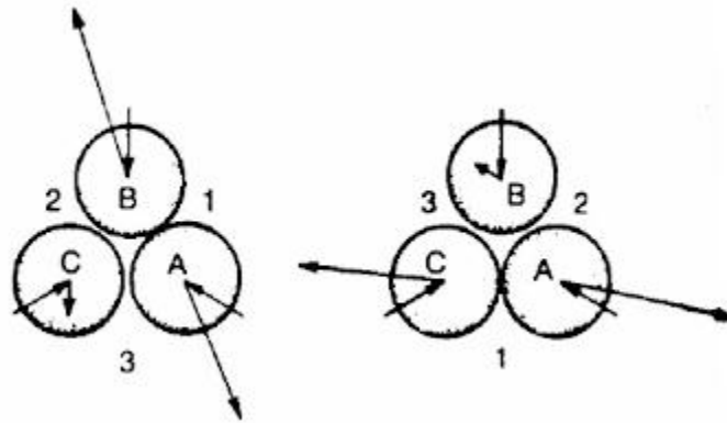
Figura V.8. Colisión triple. El comportamiento final depende críticamente de qué partículas chocan primero, de modo que el resultado depende de manera discontinua de la situación inicial.
