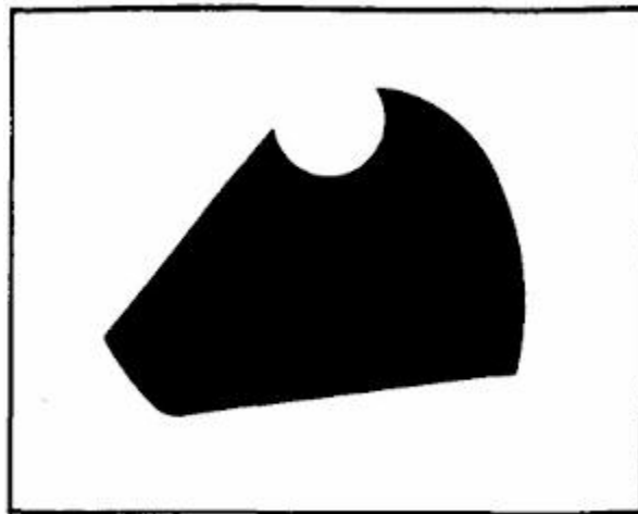
Figura IV. 1. Representación muy esquemática de un conjunto recursivo. 8
