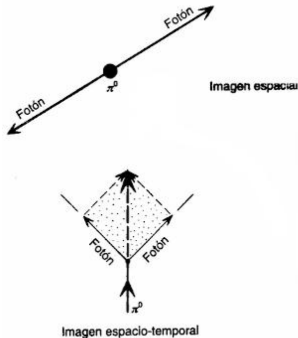
Figura V.36. Un mesón \pi^0 con masa se desintegra en dos fotones sin masa. La imagen espacio-temporal muestra cómo el cuadri-vector energía-momento se conserva: el cuadri-vector del mesón \pi^0 es la suma de los cuadri-vectores de los dos fotones sumados según la ley del paralelogramo (representado sombreado).
