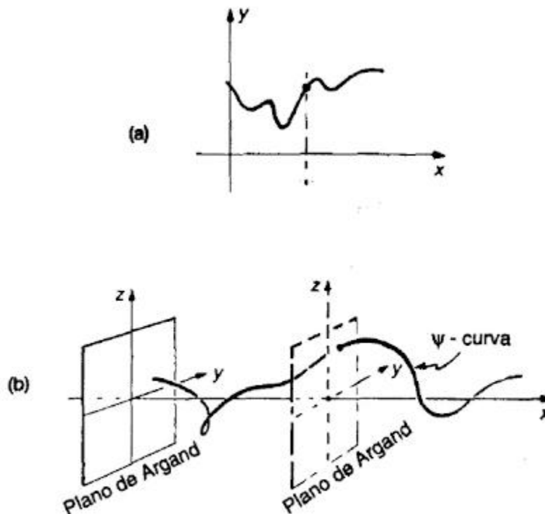
Figura VI. 10. (a) Gráfica de una función real de una variable real x .
