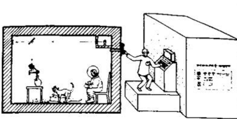
Figura VI.33. El gato de Schrödinger con aditamentos.
