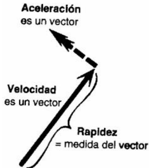
Figura V.4. Velocidad, celeridad y aceleración.
