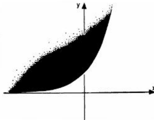
Figura IV.5. El conjunto definido por la relación exponencial y > e debería estar también entre los "recursivos".
