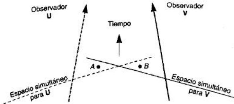
Figura VII.1 ¿Puede el tiempo "fluir" realmente? Para un observador U, B puede estar en el pasado "fijo" mientras que A está todavía en el futuro "incierto". El observador V mantendrá la opinión contraria.
