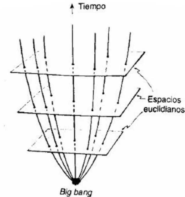
Figura VII.9. Representación espacio-temporal de un universo en expansión con secciones espaciales euclidianas (se muestran dos dimensiones espaciales).
