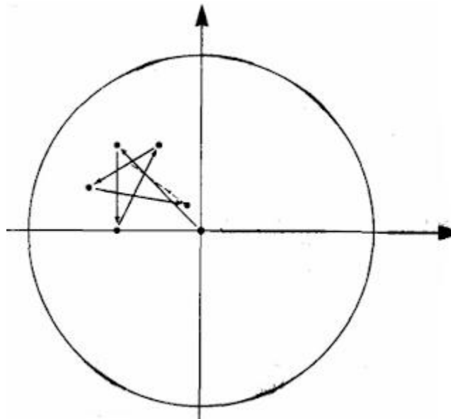
Figura III. 12. Una secuencia de puntos en el plano de Argand está acotada si existe algún círculo fijo que contiene todos los puntos.
