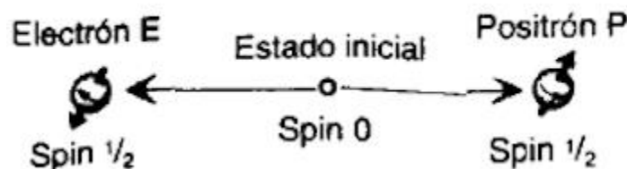
Figura VI.30. Una partícula de spin cero se desintegra en dos partículas de spin 1/2, un electrón E y un positrón P. La medida del spin de una de las partículas de spin U fija en apariencia instantáneamente el estado de spin de la otra.
