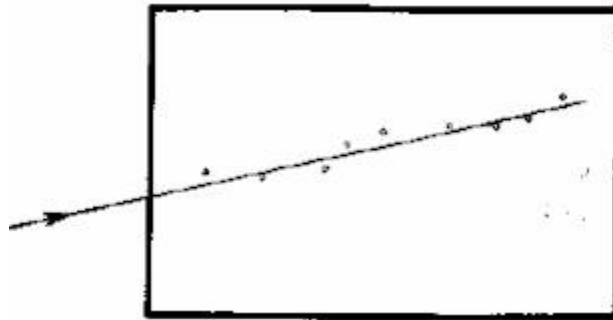
Figura VIII.7. Una partícula cargada que entra en una cámara de niebla de Wilson y provoca la condensación de una cadena de gotas.
