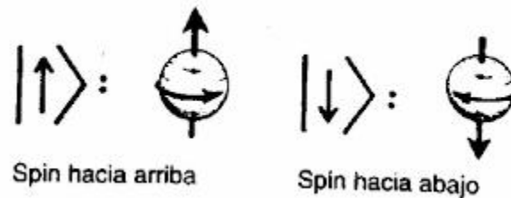
Figura VI.24. Una base para los estados de spin de un electrón consta de sólo dos estados. Éstos pueden tomarse como spin hacia arriba y spin hacia abajo.
