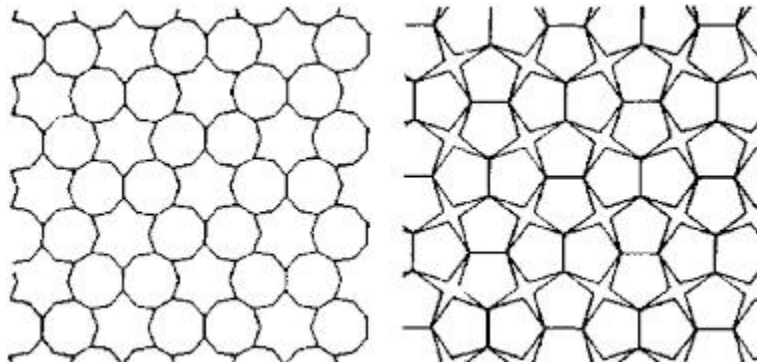
Figura IV. 7. Dos ejemplos de teselaciones periódicas del plano, de dos formas cada una.
