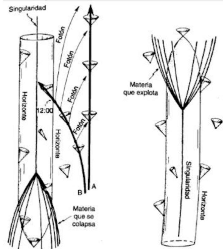
Figura VII.13 (izquierda). Diagrama espacio- tiempo que representa el colapso de un agujero negro. El radio de Schwarzschild figura marcado como "Horizonte". Figura VII.14 (derecha). Hipotética configuración espacio-tiempo: un agujero blanco que finalmente explota en materia; el inverso en el tiempo del diagrama de la figura VII.13.
