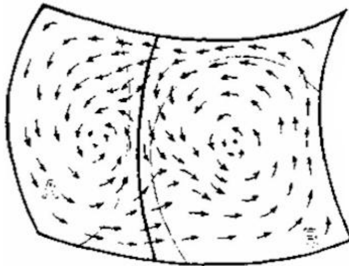
Figura VIII.5. El "flujo hamiltoniano" del contenido de la caja de Hawking (compárese con figura V. 11). Las líneas de flujo que cruzan de A a B representan el colapso en un agujero negro, y las que cruzan de B a A representan la desaparición de un agujero negro por evaporación.
