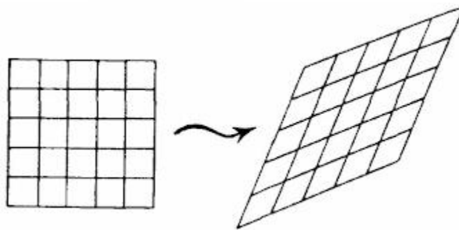
Figura V.20. Movimiento de Poincaré en dos dimensiones espacio-temporales.
