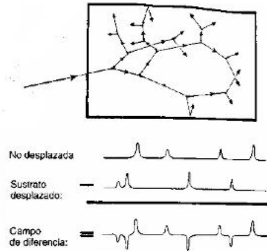
Campos gravitacionales (altamente esquemáticos) de partículas
