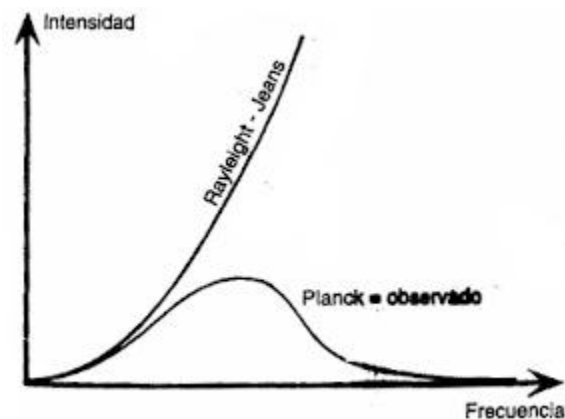
Figura VI. 2 Las discrepancias entre la intensidad de la radiación calculada clásicamente Rayleigh-Jeans— y observada para un cuerpo caliente —"cuerpo negro"— llevaron a Planck a los inicios de la teoría cuántica.
