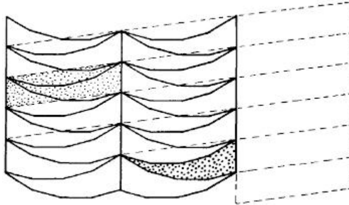
Figura IV. 8. Una teselación periódica, ilustrada en relación con su paralelogramo periodo.
