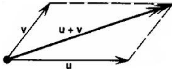
Figura V.6. Ley del paralelogramo para la suma vectorial.
