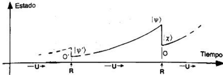
Figura VIII.1. Evolución temporal de un vector de estado: evolución unitaria suave U (según la ecuación de Schrödinger) interrumpida por la reducción discontinua R del vector de estado.
