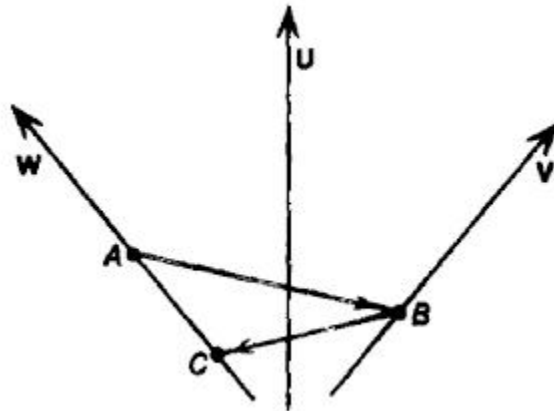
Figura V.32. Si V está equipado con un dispositivo que envía señales más rápidas que la luz, idénticas al de W, pero apuntando en la dirección opuesta, puede ser utilizado por W para enviar un mensaje a su propio pasado.
