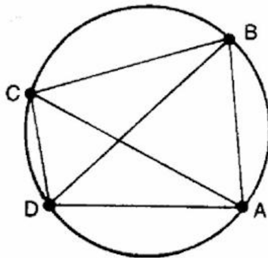
Figura V.3. El teorema De Tolomeo.
