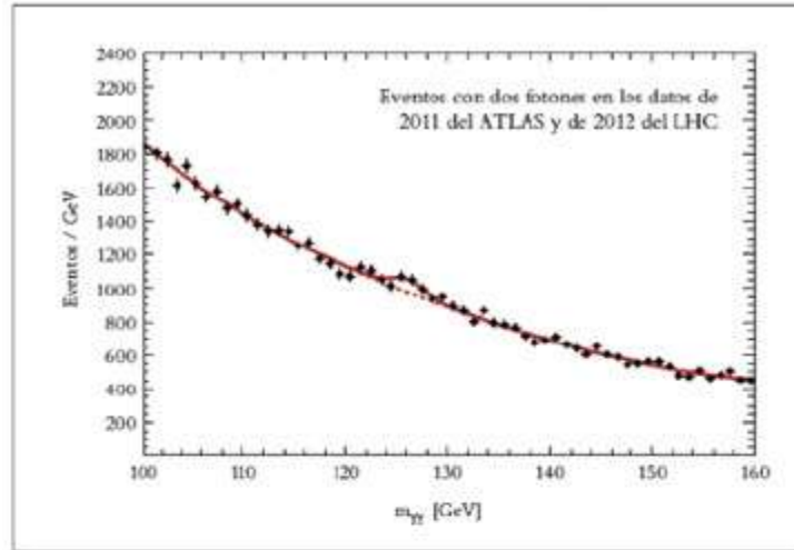
Los datos producidos y analizados en la búsqueda del Higgs en el LHC. Estas gráficas muestran el número de eventos que producen dos fotones de alta energía, donde la energía total de los fotones va desde 100 a 160 GeV, en los datos de 2011-2012 de ATLAS y CMS. Las líneas de puntos marcan la predicción sin ningún bosón de Higgs; la línea continua incluye un Higgs con una masa de 126,5 GeV (ATLAS) o 125,3 GeV (CMS). © CERN
