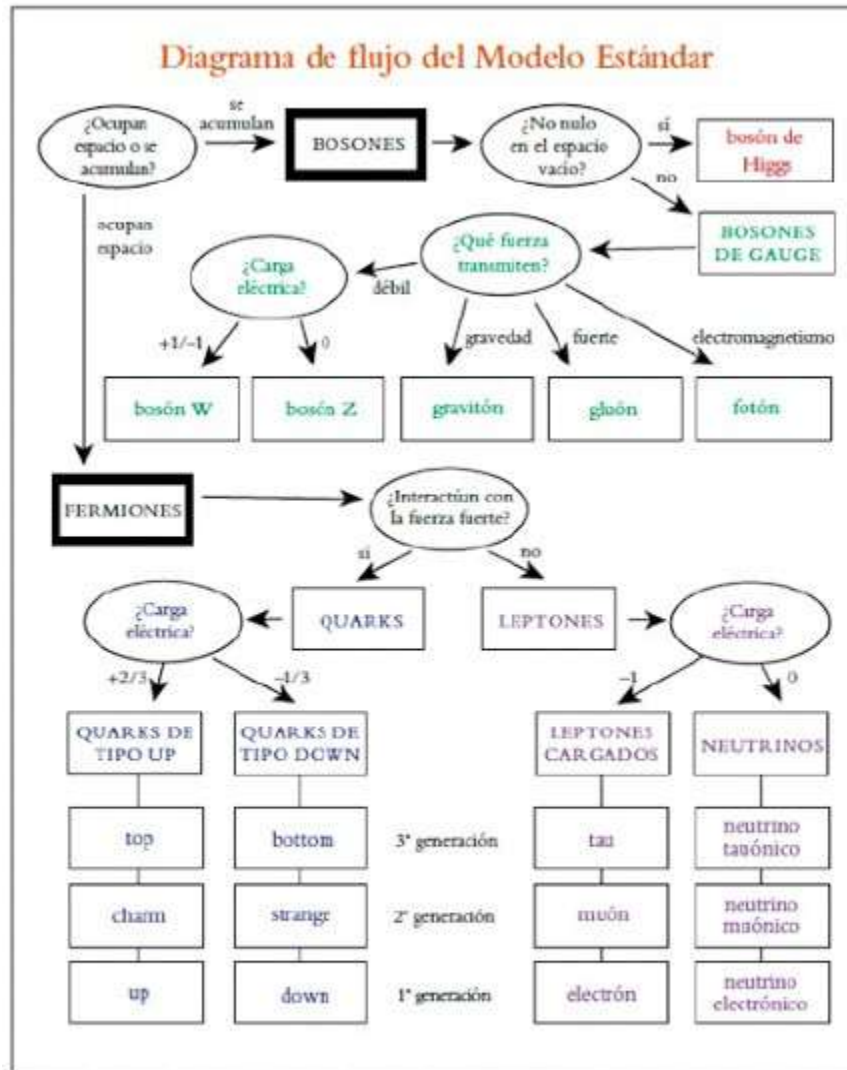
Diagrama de flujo que ilustra las partículas elementales del Modelo Estándar. Esta es la versión moderna de la tabla periódica de los elementos. Los quarks aparecen en azul, los leptones en morado, los bosones de gauge en verde y el bosón de Higgs en rojo. SEAN CARROLL.
