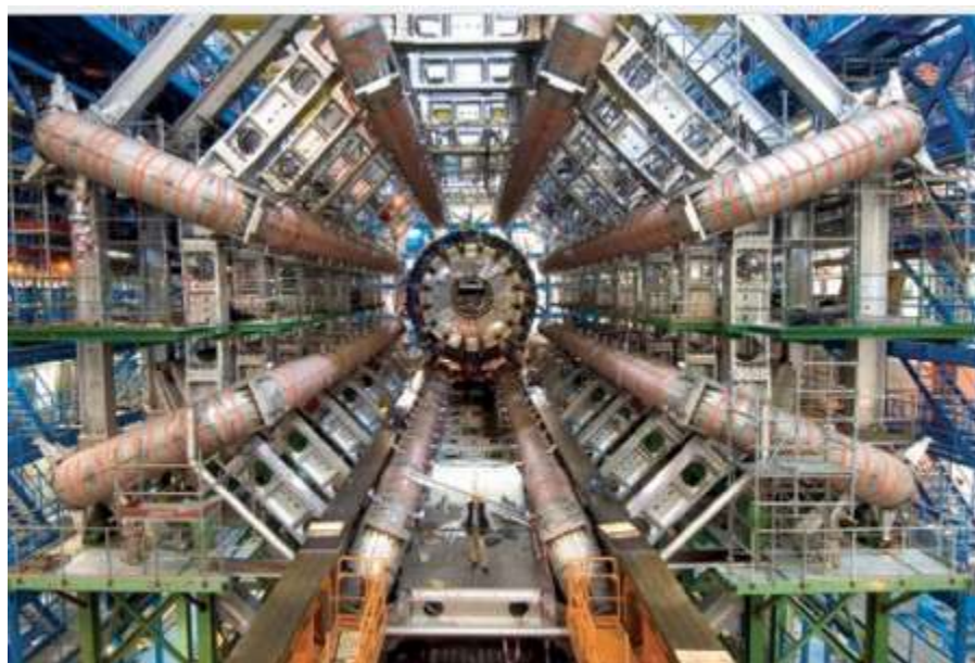
El detector ATLAS en construcción. Fíjese en la persona que aparece en la zona inferior del centro de la imagen. Las ocho tuberías gigantes son imanes, que se utilizan para desviar a los muones y así poder medir sus energías. © CERN
