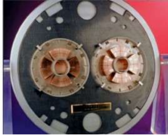
Sección transversal de los imanes dipolares del LHC. Por los dos tubos de los haces se mueven los protones en direcciones opuestas. © CERN
