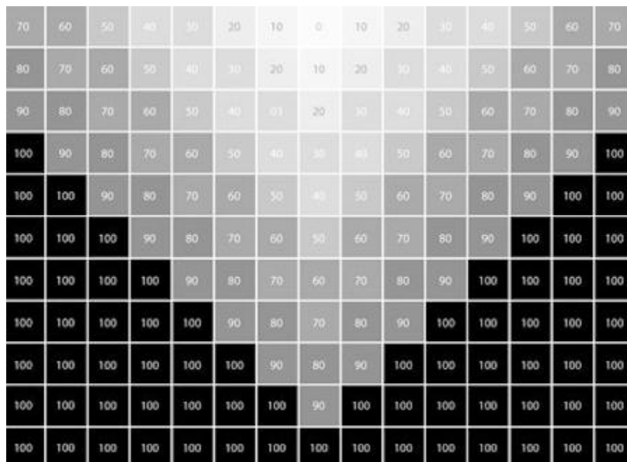
Figura 3.8a. Cada fila registra el valor del inflatón en un instante de tiempo desde la perspectiva de alguien que está fuera. Las filas más altas corresponden a momentos más tardíos. Las columnas denotan posiciones en el espacio. Una burbuja es una región del espacio que deja de inflarse debido a una caída del valor del inflatón. Las
