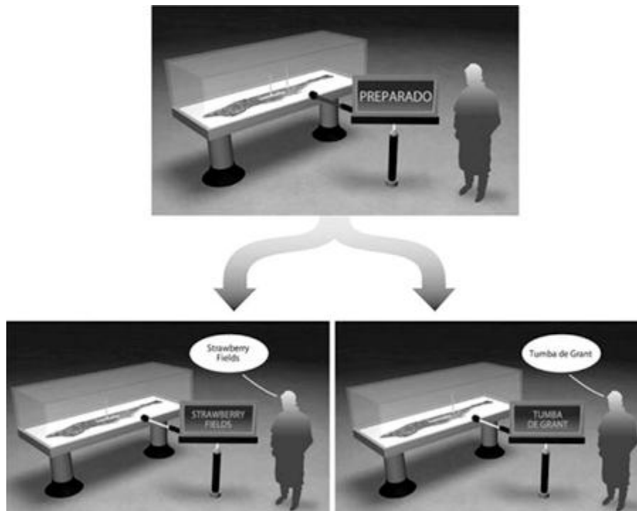
Figura 8.12. En la aproximación de Everett, la medida de una partícula cuya onda de probabilidad tiene dos picos da ambos
