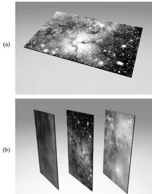
Figura 5.3. (a) En el escenario mundobrana se imagina que lo que tradicionalmente hemos pensado que es el cosmos entero reside en una brana tridimensional. Para facilitar la visualización, suprimimos una dimensión y mostramos el mundobrana como si tuviera dos dimensiones espaciales; también mostramos sólo un fragmento finito de branas que pueden extenderse infinitamente lejos. (b) La extensión
