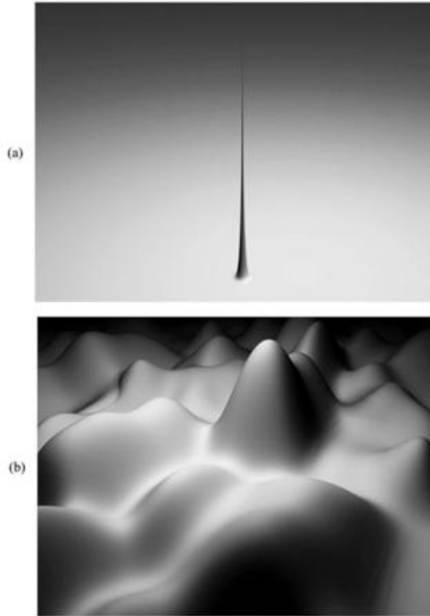
Figura 8.5. (a) La onda de probabilidad para un objeto macroscópico es generalmente una onda estrecha y puntiaguda. (b) La onda de probabilidad para un objeto microscópico, digamos, una única partícula, está normalmente muy extendida.
