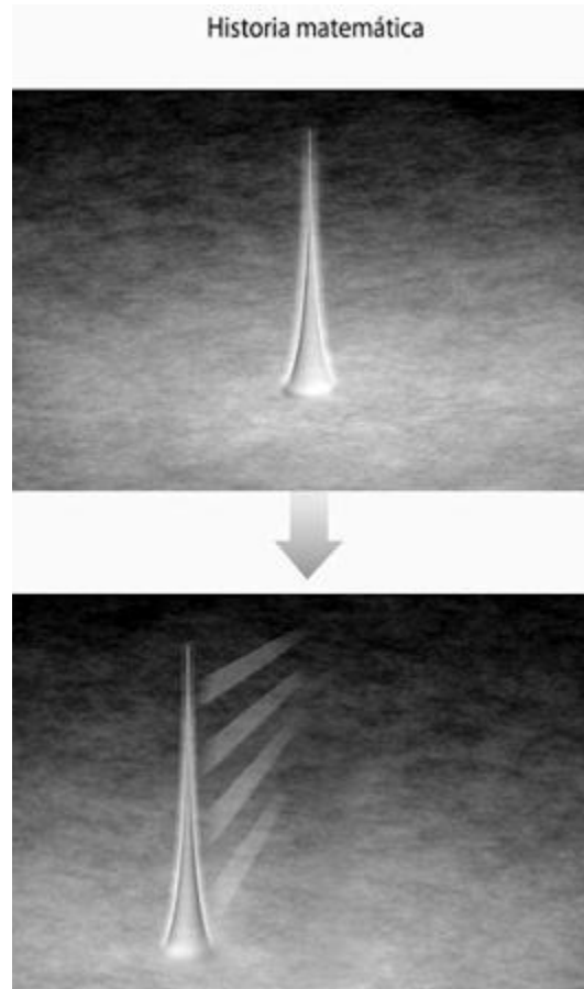
Figura 8.15. (a) El mismo tipo de evolución matemática que en la Figura 8.14a, pero con la onda de probabilidad del electrón con el pico en la tumba de Grant.
