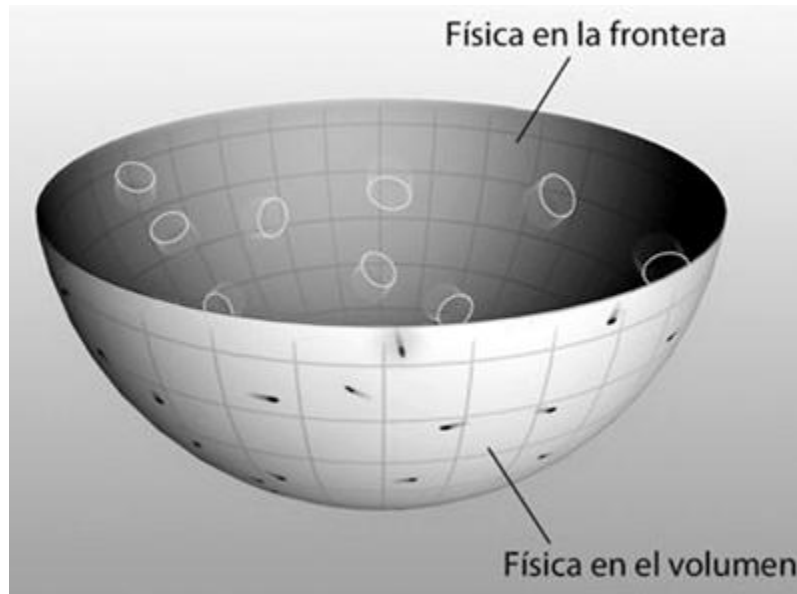
Figura 9.5. Una ilustración esquemática de la dualidad entre teoría de cuerdas que actúa en el interior de un espacio-tiempo particular y teoría cuántica de campos en la frontera de dicho espacio-tiempo.
