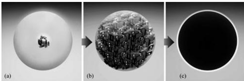
Figura 9.3. (a) Una variedad de objetos que almacenan información, situada dentro de una región bien definida del espacio. (b)
