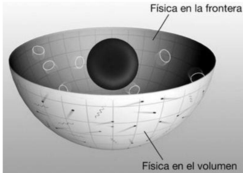
Figura 9.6. La equivalencia holográfica aplicada a un agujero negro en el volumen del espacio-tiempo da un baño caliente de partículas y radiación en la frontera de la región.
