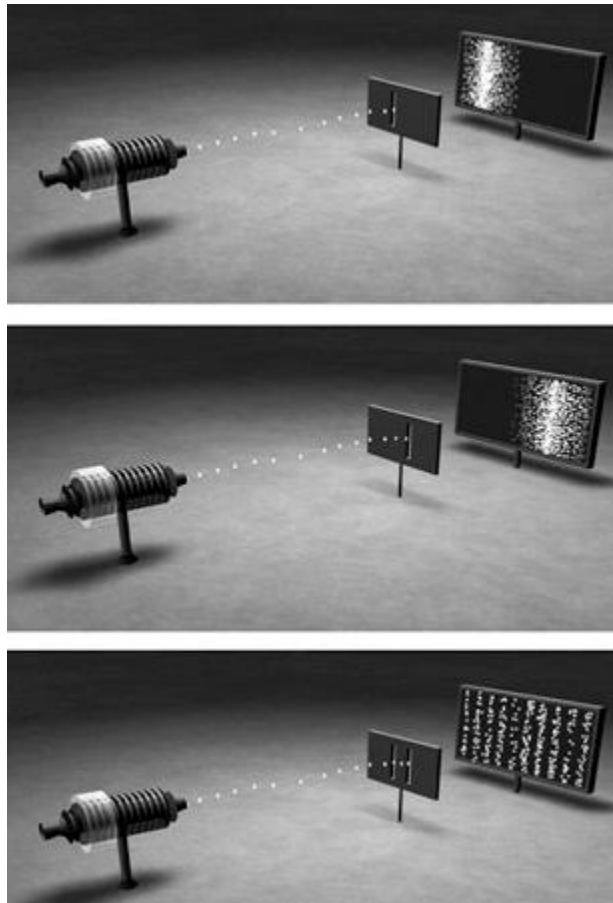
Figura 8.2. (a) Los datos obtenidos cuando se disparan los electrones y sólo la rendija izquierda está abierta. (b) Los datos obtenidos cuando se disparan los electrones y sólo la rendija derecha está
