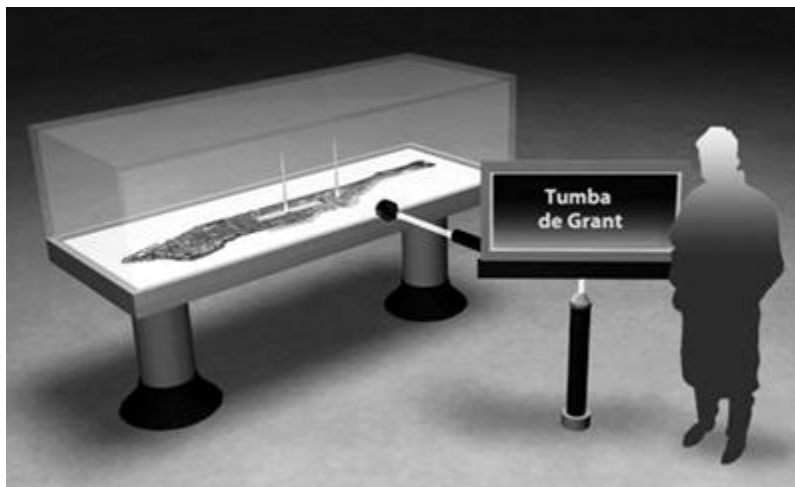
Figura 8.10. La onda de probabilidad de un electrón tiene picos en dos localizaciones. La linealidad de la ecuación de Schrödinger sugiere que una medida de la posición del electrón daría una amalgama confusa de ambas localizaciones.
