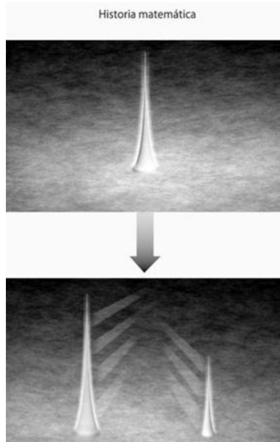
Figura 8.18. (a) Una ilustración esquemática de la evolución, dictada por la ecuación de Schrödinger, de la onda de probabilidad combinada para todas las partículas que le constituyen a usted y su aparato de medida, cuando usted mide la posición de un electrón. La propia onda de probabilidad del electrón tiene picos en dos localizaciones, pero con alturas desiguales.
