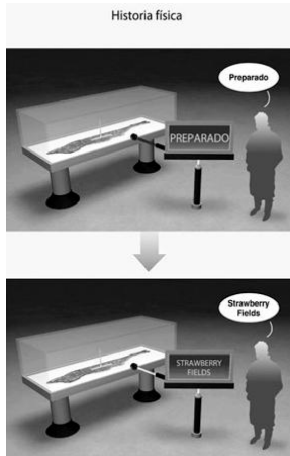
Figura 8.15. (b) La correspondiente historia física, o experimental.
