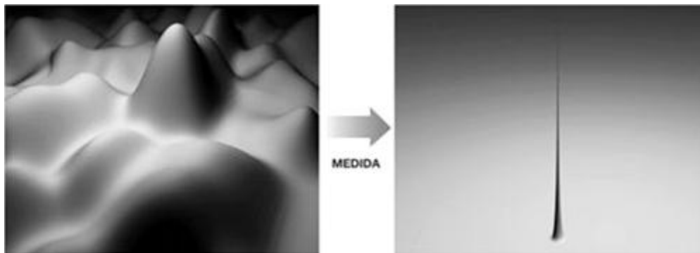
Figura 8.6. La aproximación de Copenhague a la mecánica cuántica imagina que cuando se mide u observa, la onda de probabilidad de una partícula colapsa instantáneamente en todas las localizaciones salvo en una. El abanico de posiciones posibles para la partícula se transforma en un resultado definido.
