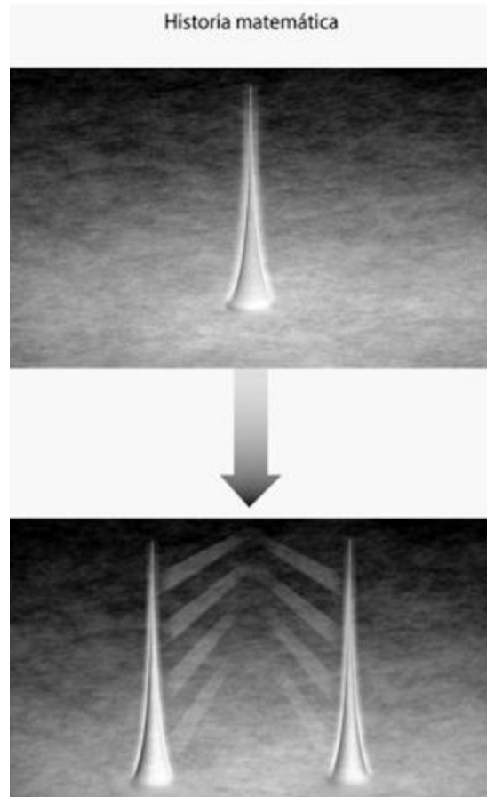
Figura 8.16. (a) Una ilustración esquemática de la evolución de la onda de probabilidad combinada de todas las partículas que le constituyen a usted y su aparato de medida, cuando se mide la posición de un electrón cuya onda de probabilidad tiene picos en dos localizaciones.
