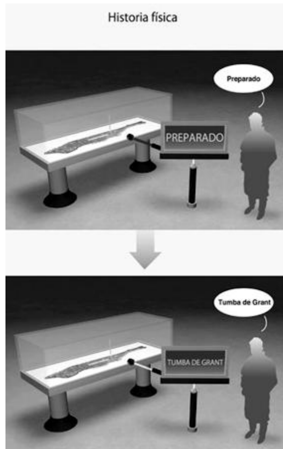
Figura 8.14. (b) La correspondiente historia física, o experimental.
