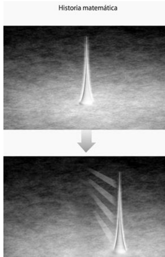
Figura 8.14. (a) Una ilustración esquemática de la evolución, dictada por la ecuación de Schrödinger, de la onda de probabilidad combinada para todas las partículas que le constituyen a usted y su aparato de medida, cuando usted mide la posición de un electrón. La propia onda de probabilidad del electrón tiene un pico en Strawberry Fields.
