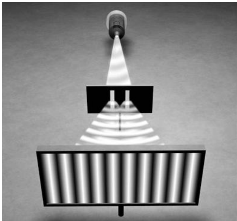
Figura 8.4. Cuando describimos el movimiento de un electrón en términos de una onda de probabilidad ondulante se explican los enigmáticos datos de interferencia.
