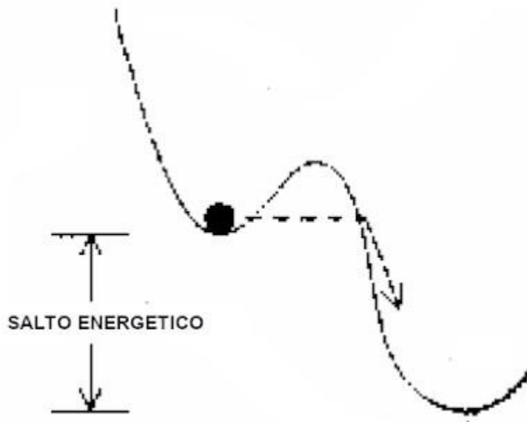
Figura 10.3. Estados de vacío falso y auténtico. Puede darse el caso de que el actual estado cuántico de espacio vacío A no sea el estado de menor energía sino que, sin embargo, esté casi estabilizado al corresponderse con una especie de valle de alta montaña. Habría entonces una pequeña probabilidad de que ese estado degenerara por el efecto túnel a un auténtico estado estable de base B. La transición entre estos estados, que se daría mediante la formación de una burbuja, liberaría una inmensa cantidad de energía.
