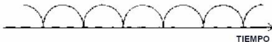
Figura 11.1. El modelo de universo cíclico. El universo muestra un pulso en tamaño de manera periódica entre estados muy densos y estados muy distendidos. Cada ciclo empieza con un gran pum y termina con un gran crujido y es aproximadamente simétrico con respecto al tiempo.
