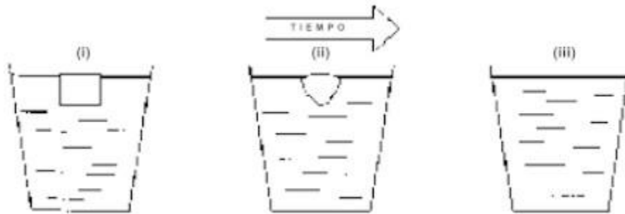
Figura 2.1. La flecha del tiempo. El cubito de hielo que se derrite, define la dirección del tiempo: el calor fluye del agua caliente al hielo frío. Una película que fuera en el sentido (iii), (ii), (i) se reconocería inmediatamente como falsa. Esta asimetría está caracterizada por una magnitud llamada entropía que aumenta conforme va fundiéndose el hielo.
