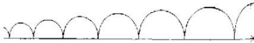
Figura 11.2. Los procesos irreversibles hacen que los ciclos cosmológicos crezcan más y más, destruyendo así el auténtico carácter cíclico.
