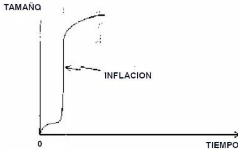
Figura 3.3. La situación inflacionaria. En tal situación, el universo da un salto súbito y grande en su tamaño al poquísimo tiempo de originarse en una explosión. La escala vertical esta tremendamente comprimida. Después de la fase inflacionaria, la expansión prosigue a un ritmo cada vez más lento, de manera parecida a la mostrada en la figura 3.2
