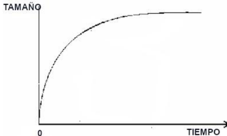
Figura 3.2. La tasa de expansión del universo se decelera progresivamente con el paso del tiempo aproximadamente como muestra la figura. En este sencillo modelo, la tasa de expansión es infinita en el punto marcado como 0 en el eje del tiempo. Es el punto que se corresponde con el gran pum
