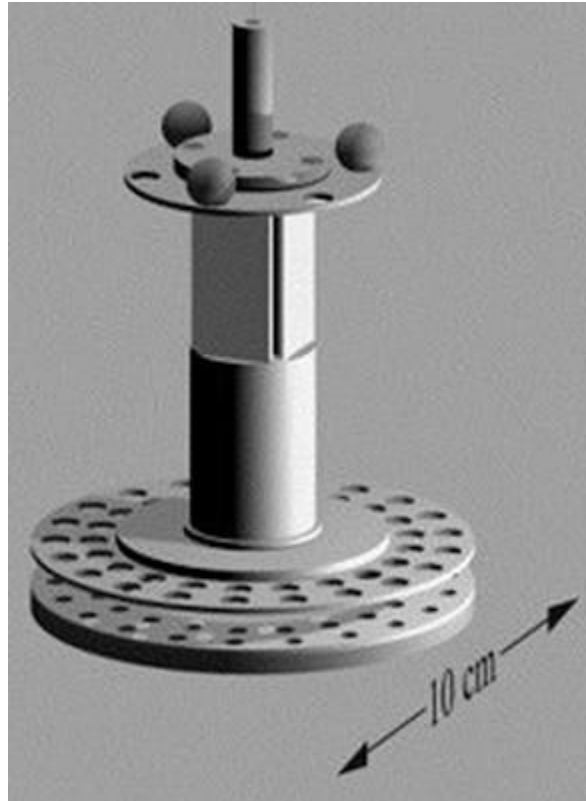
Figura 76. El aparato del experimento Eöt-Wash. Un anillo se encuentra suspendido sobre dos discos. Los agujeros del anillo y de los discos garantizan que el anillo no girará si se cumple la ley del cuadrado del inverso de Newton. Las tres esferas que hay cerca de la parte superior del aparato se usan para calibrarlo.
