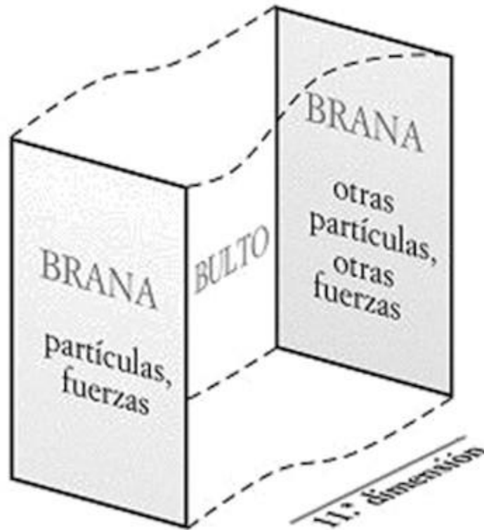
Figura 72. Dibujo esquemático del mundo brana de Hořava-Witten.
