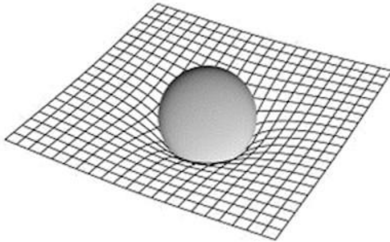
Figura 39. Un objeto con masa distorsiona el espacio que lo rodea, creando así un cuerpo gravitatorio.
