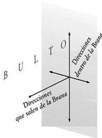
Figura 25. Una brana es una superficie de dimensión inferior con direcciones sobre ella y direcciones que parten de ella, adentrándose en el bulto de dimensión superior.
