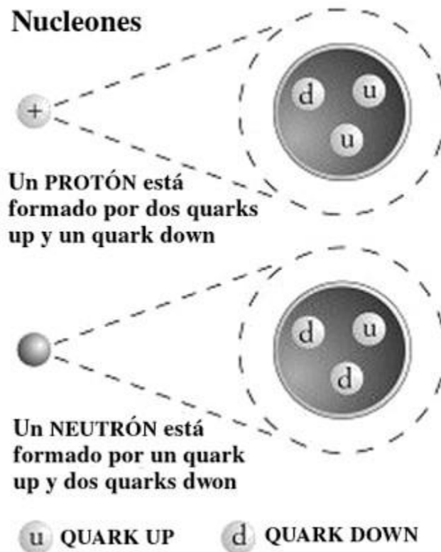
Figura 31. El protón y el neutrón están compuestos de partículas más elementales, llamadas quarks, unidas entre sí por la fuerza fuerte.
