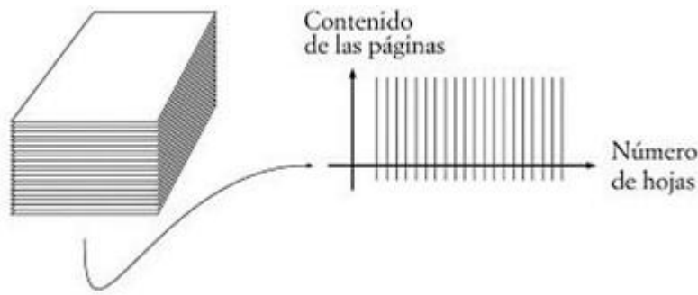
Figura 8. Un libro tridimensional está hecho de hojas bidimensionales.
