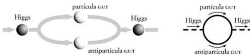
Figura 61. La contribución virtual a la masa de la partícula de Higgs proveniente de las partículas pesadas en una gran teoría unificada (GUT). La partícula de Higgs puede convertirse en partículas virtuales pesadas (con una masa de la gran teoría unificada), que luego vuelven a convertirse, a su vez, en una partícula de Higgs. Esto se ilustra por medio de un esquema a la izquierda, y con un diagrama de Feynman, a la derecha.
