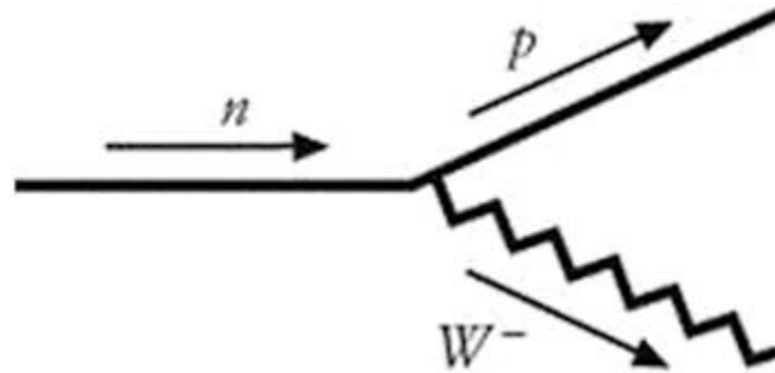
Figura 49. La interacción con un bosón gauge W^- transforma un neutrón en un protón (y un quark down contenido en el neutrón en un quark up contenido en el protón).
