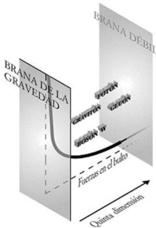
Figura 83. Las fuerzas no gravitatorias pueden estar también en el bulto. En ese caso, las fuerzas pueden unificarse a altas energías.
