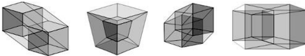
Figura 14. Proyecciones de un hipercubo.
