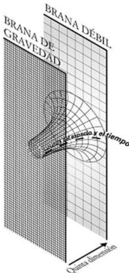
Figura 82. El tamaño aumenta (y la masa y la energía disminuyen) cuando nos alejamos de la Brana de Gravedad y nos aproximamos a la Brana Débil.
