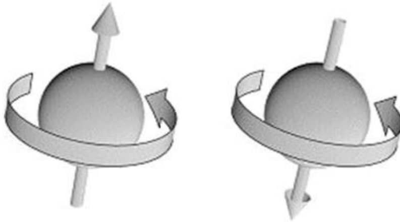
Figura 48. Los quarks y los leptones pueden ser dextrógiras o levógiras.
