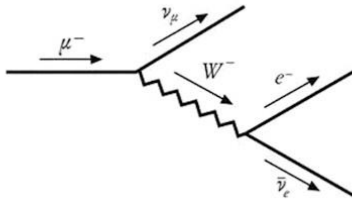
Figura 53. En la desintegración del muón, éste se convierte en un neutrino muón y un bosón gauge virtual W^- , que se convierte a su vez en un electrón y un antineutrino electrón.
