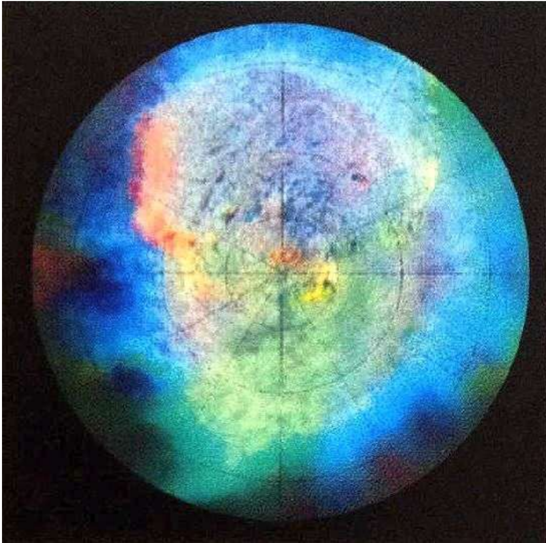
Tritón visto justo sobre su polo. Las diferencias de color se han exagerado en gran medida. Cedida por USGS/NASA.
