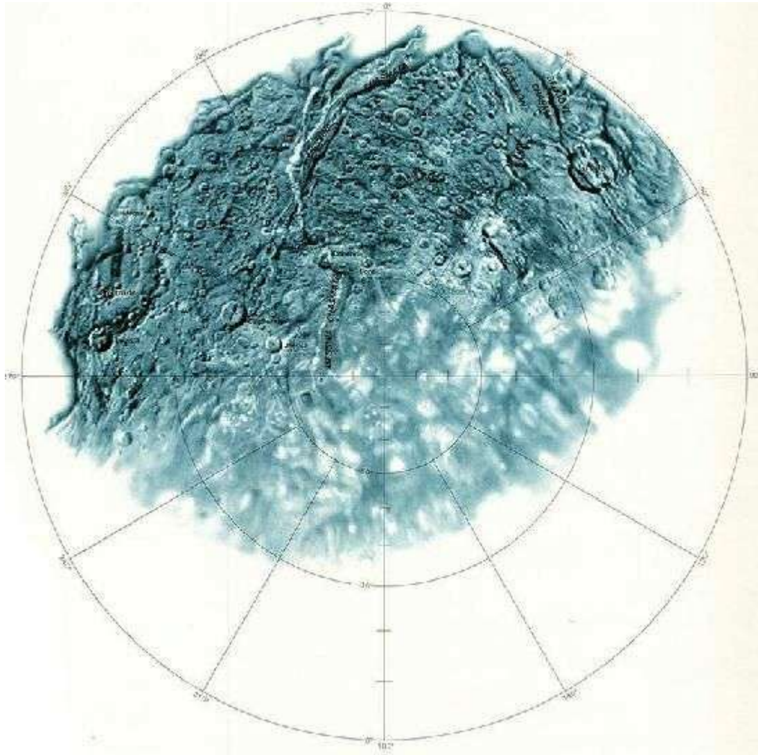
Proyección del polo sur de Titania, otra de las lunas de Urano. Mapa en relieve sombreado de USGS.
