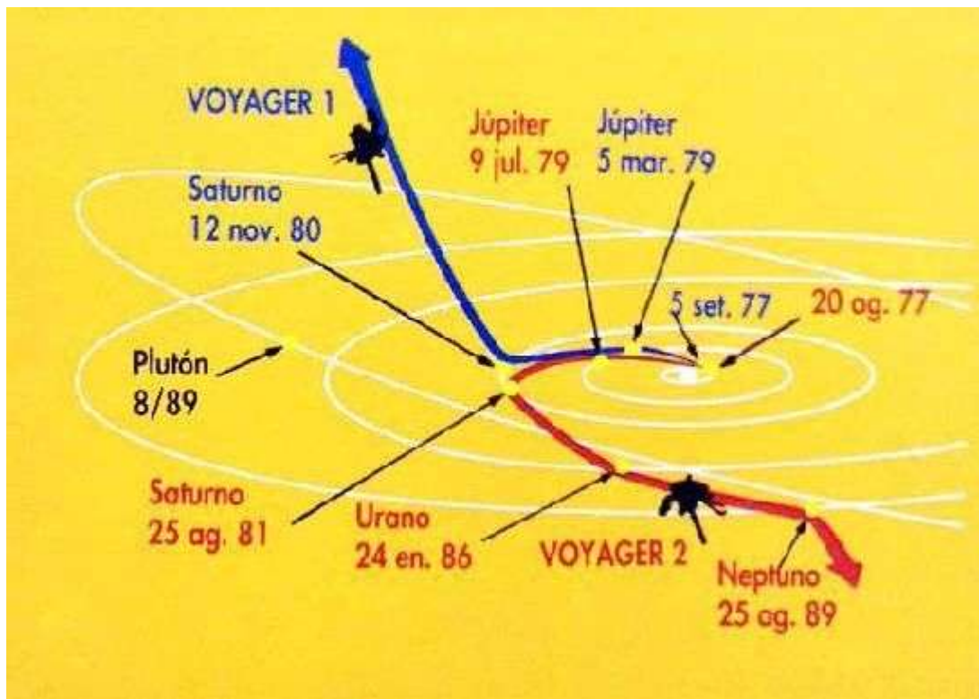
Trayectorias de las dos naves Voyager. Cedita por JPL/NASA.
