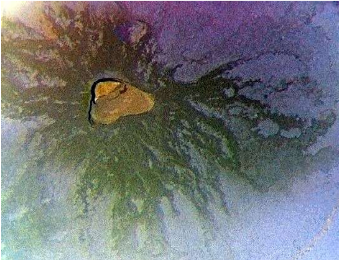
Construcción volcánica Maasaw Patera, en Ío. Corrientes de lava, quizá de azufre fundido, surgieron de su caldera en un determinado momento. Datos del Voyager, cedida por USGS/NASA.
