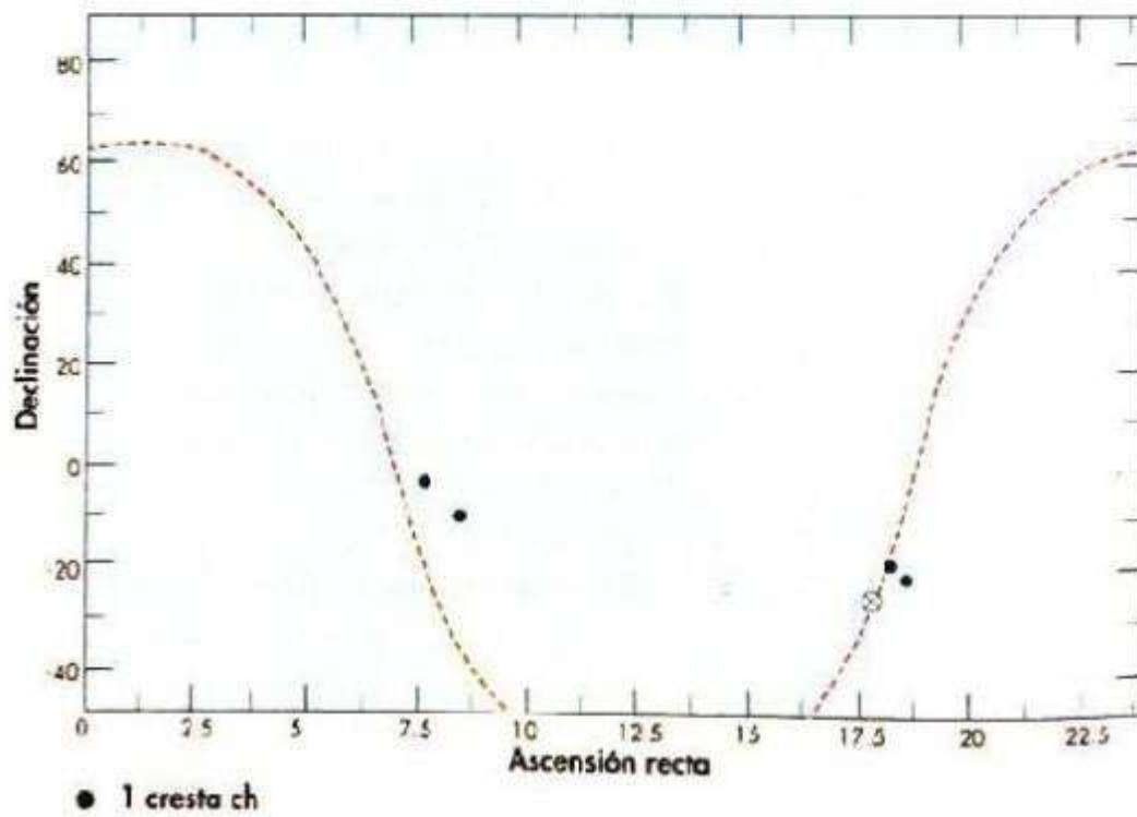
Distribución de las fuentes de radio META por el cielo. La declinación y la ascensión recta son las coordenadas de latitud y longitud del
