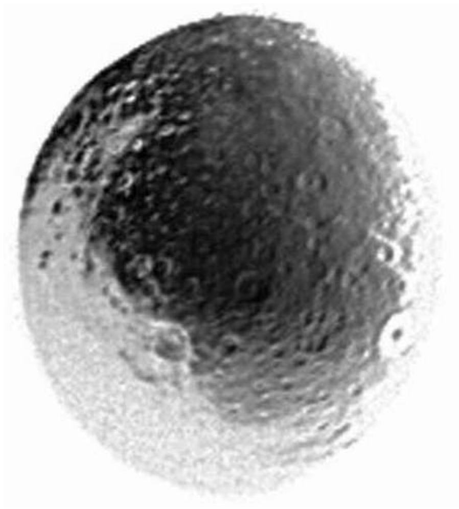
Japeto vista desde el Voyager. Imagen en negativo cedida por USGS/NASA.
