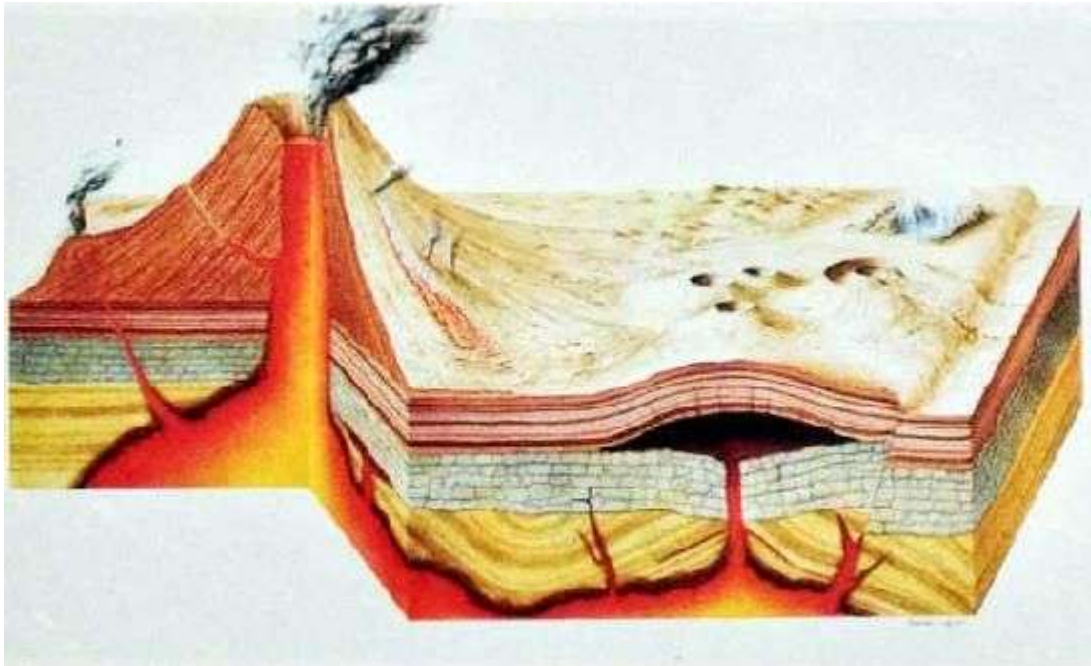
Sección de un volcán drenando los yacimientos subterráneos de roca líquida. Pintura de Kazuaki Iwasaki.
