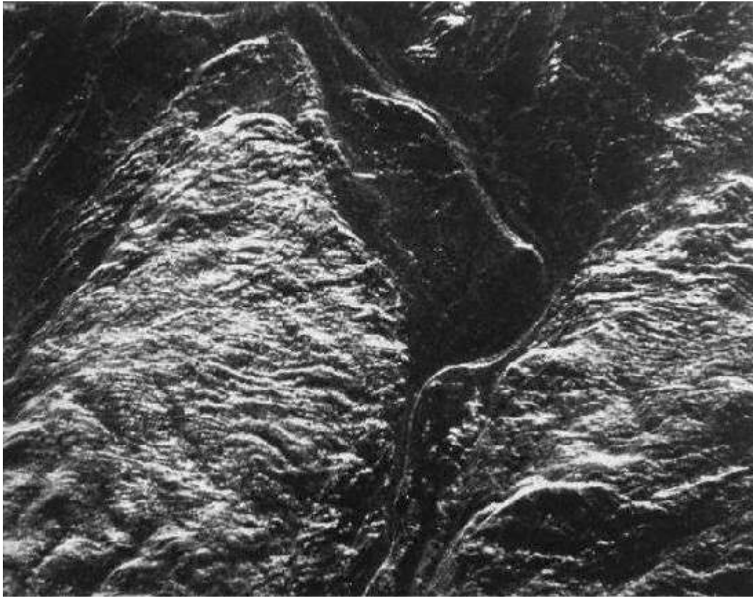
Sinuoso canal al norte de las montañas Freyja, de Venus. Datos de la sonda Magallanes, cedida por JPL/NASA.
