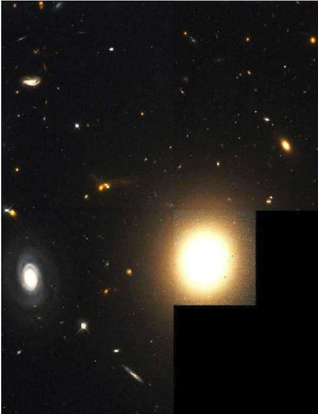
El universo de galaxias. Esta espectacular fotografía, obtenida por el telescopio espacial Hubble, muestra la periferia del cúmulo galáctico
