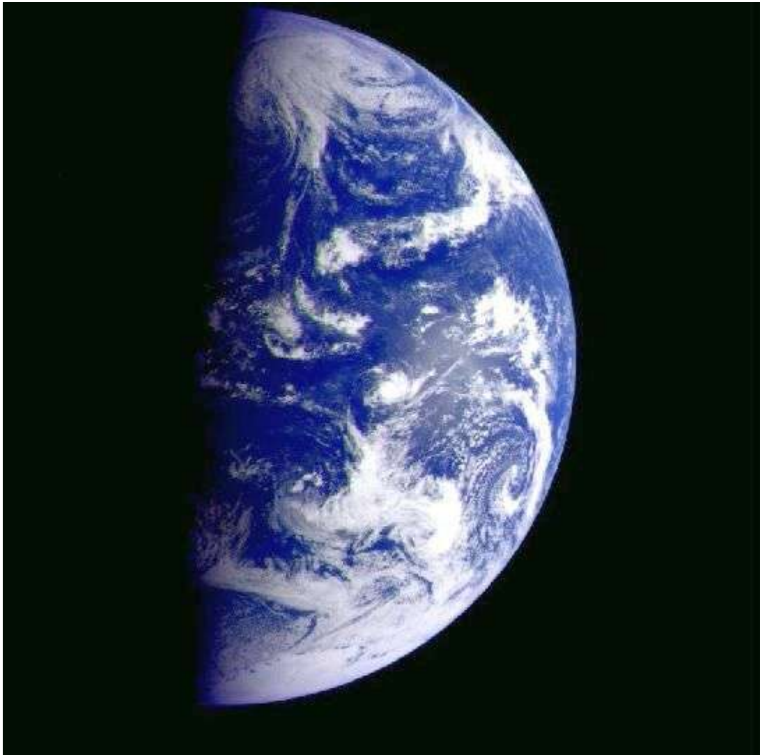
La Tierra desde la nave Galileo. No hay indicio de vida. Cedida por JPL/NASA.
