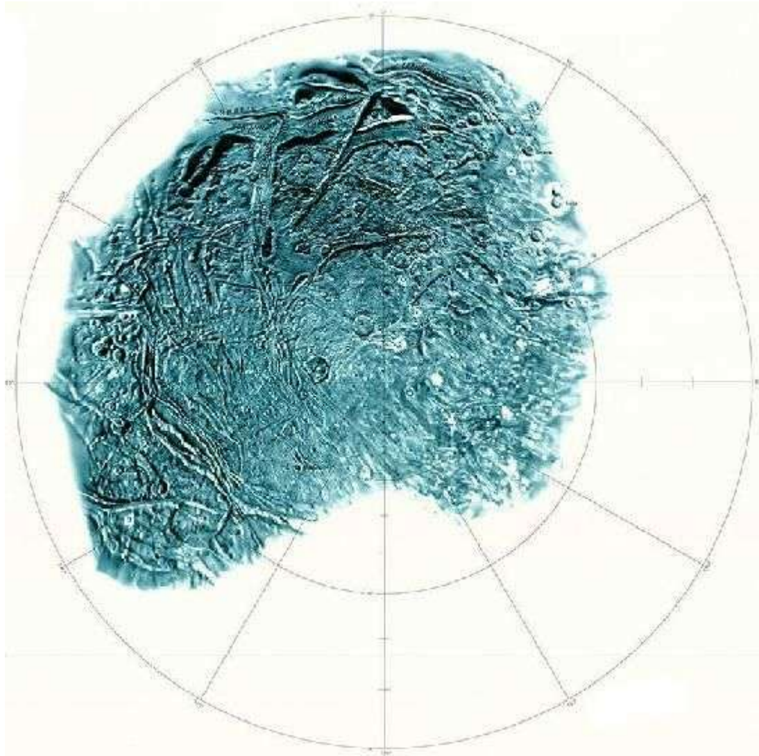
Proyección del polo sur de Ariel, una de las lunas de Urano. Mapa en relieve sombreado de USGS.
