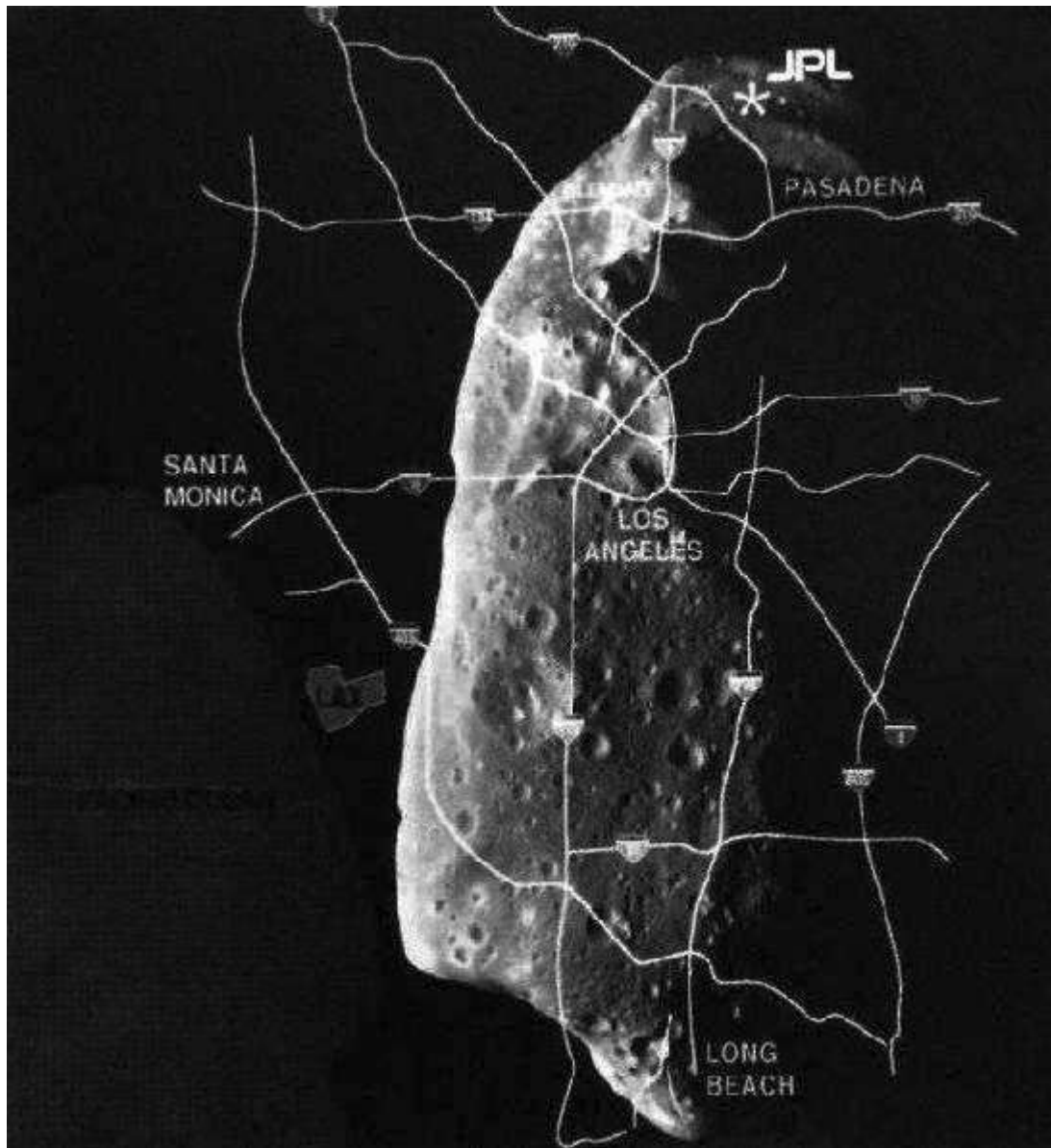
Gaspra comparado con el sistema de autopista de Los Ángeles.
