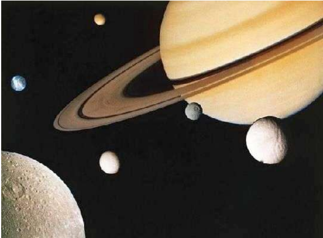
Fotomontaje de Saturno y algunas de sus lunas. Titán aparece en la parte superior.
