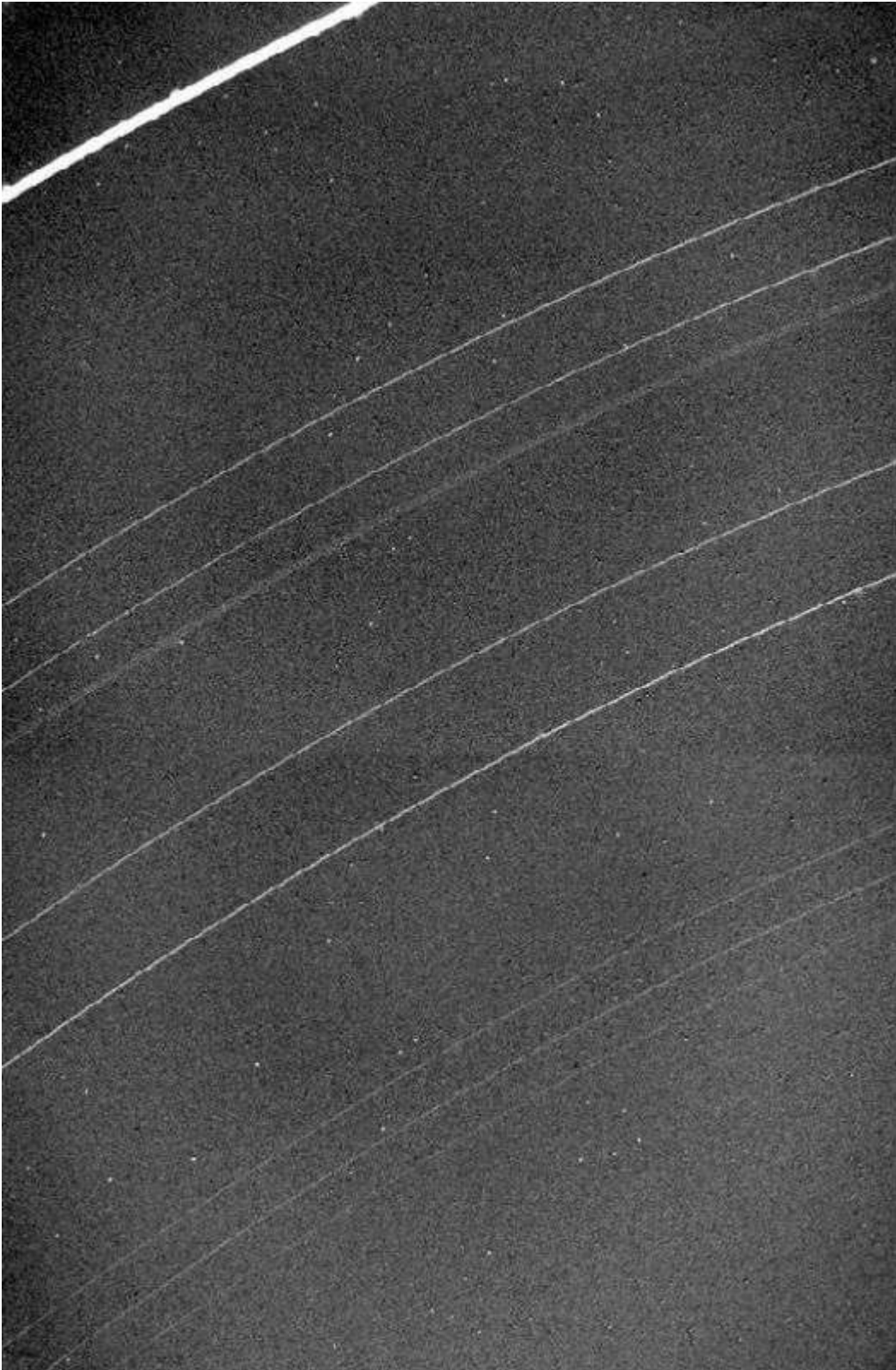
Otra panorámica de los anillos de Urano. El más ancho, \epsilon , tiene menos de cien kilómetros de anchura. Algunos de los restantes miden
