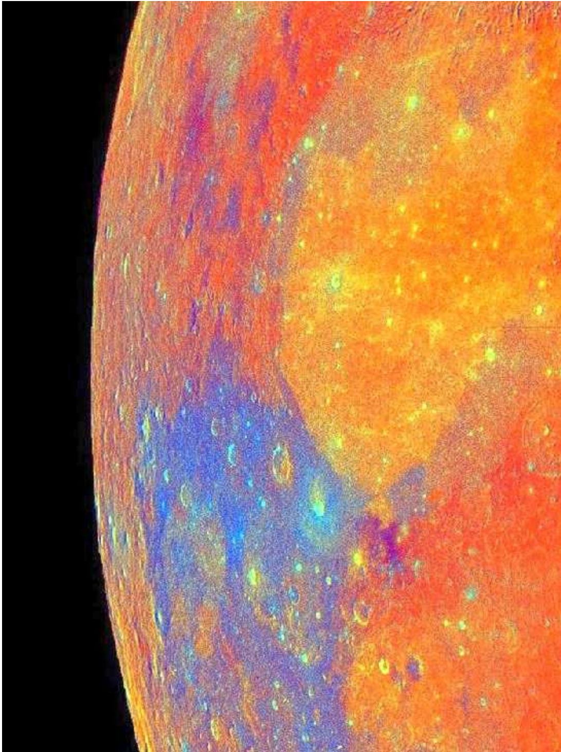
Los cráteres salpican el paisaje lunar en esta imagen de color falso tomada por la nave Galileo. Cedida por JPL/NASA.
