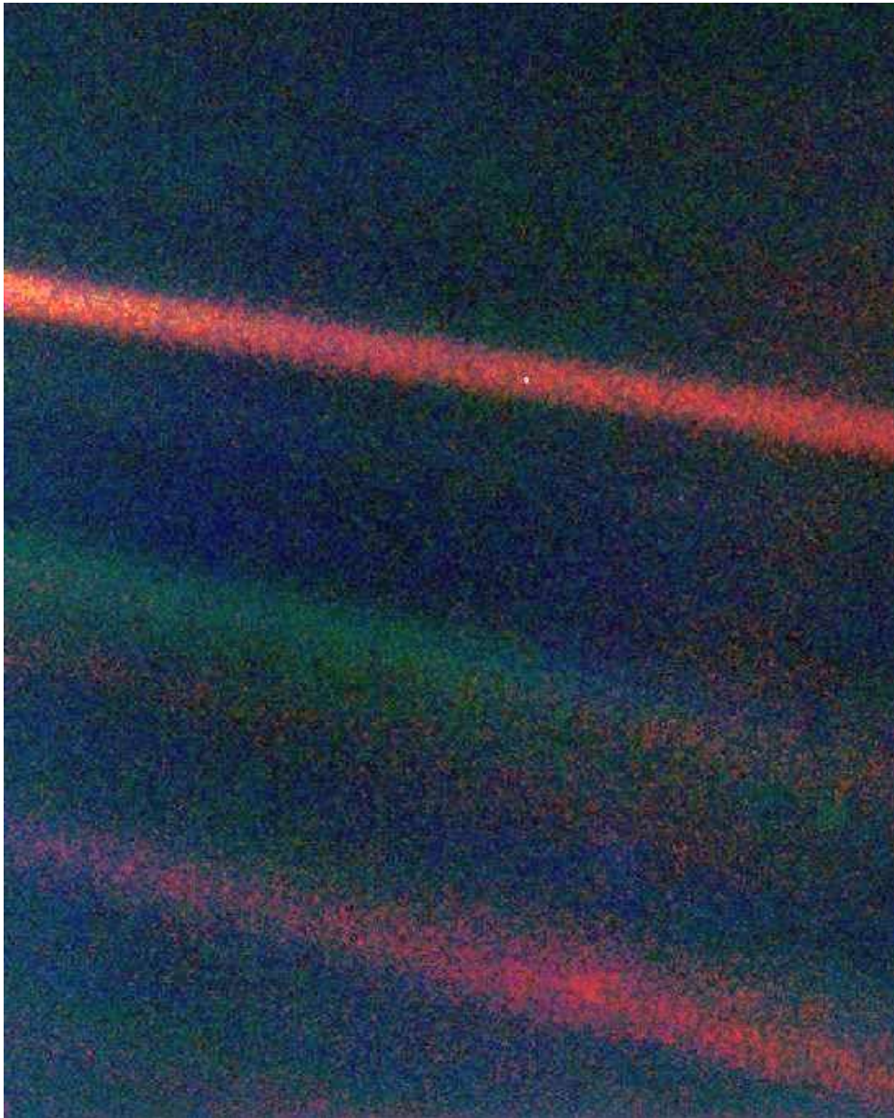
La Tierra, un punto azul pálido en un rayo de sol, fotografiado por el Voyager 2 desde más allá de la órbita de Neptuno.
