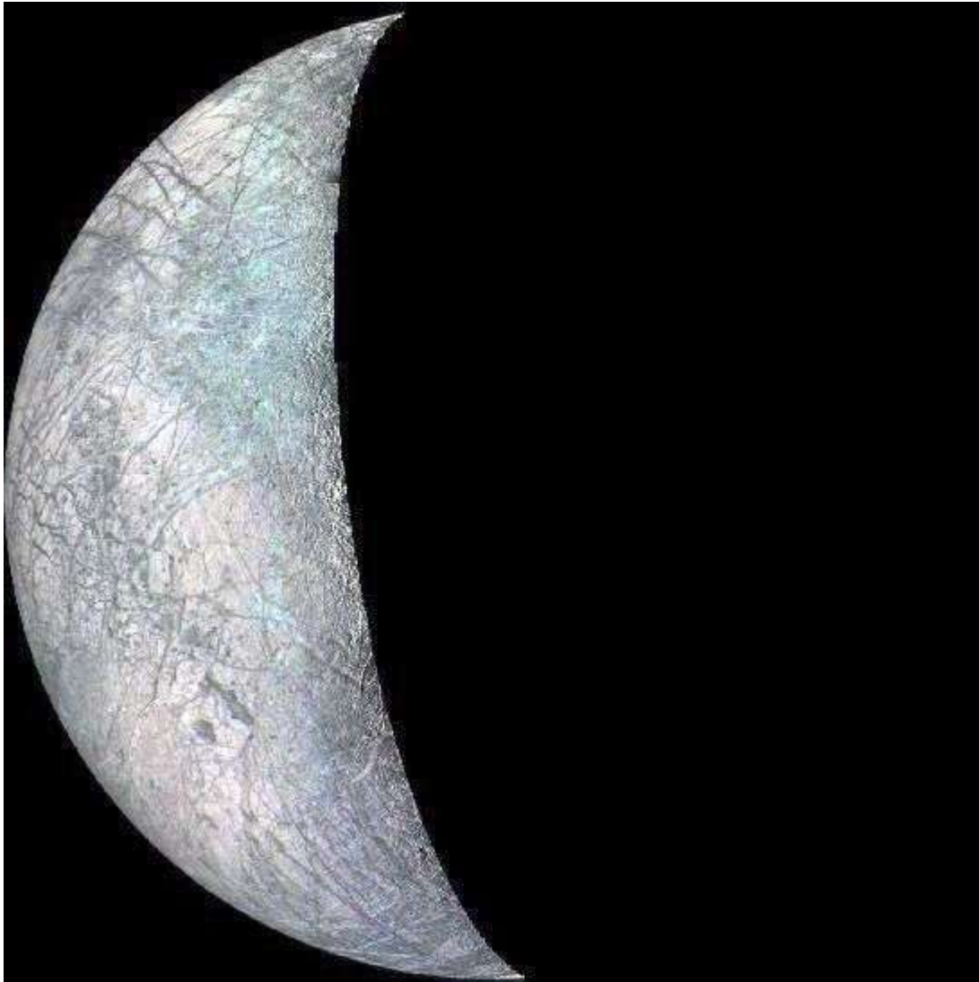
Fotomosaico de una porción de la superficie de Europa vista por el Voyager. Cedido por USGS/NASA.
