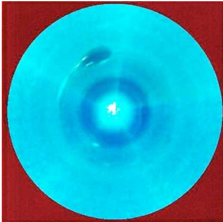
Proyección del polo sur de Neptuno. Cedida por JPL/NASA.
