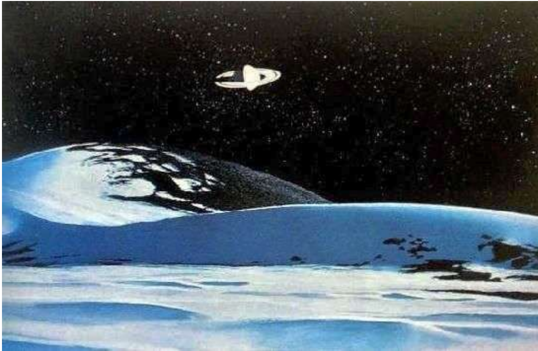
Concepción artística de la superficie de Japeto, un extraño mundo de hielo y materia orgánica compleja, en una órbita exterior a Titán. Saturno se vislumbra en su cielo. Pintura de Ron Miller.
