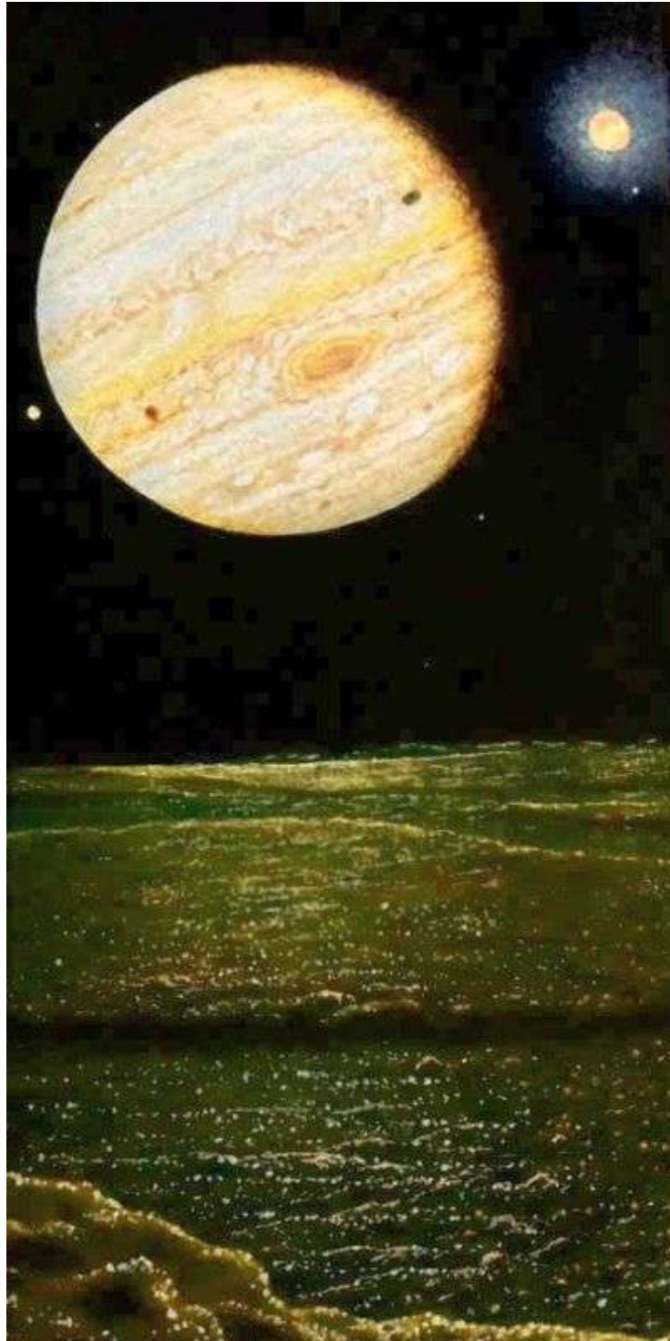
Júpiter visto desde la superficie de Europa. La luna que aparece a la derecha, rodeada de una nube de gases en escape, es Ío. Algunos científicos creen que existe un océano subterráneo de agua en Europa. Pintura de Don Davis.
