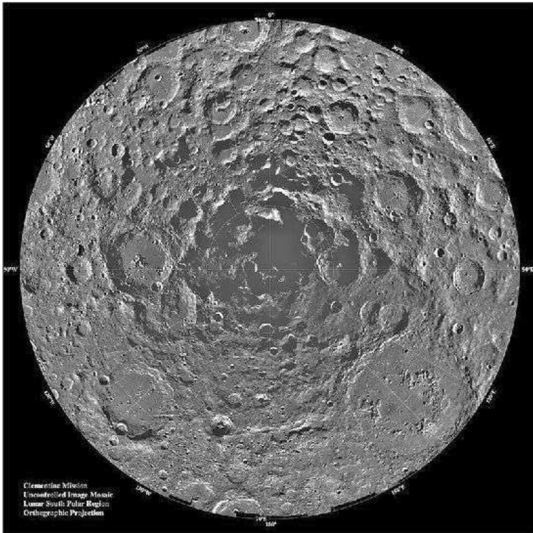
La vapuleada y devastada región del polo sur de la Luna. Fotomosaico de la misión Clementine, cedida por Naval Research Laboratory y USGS.
