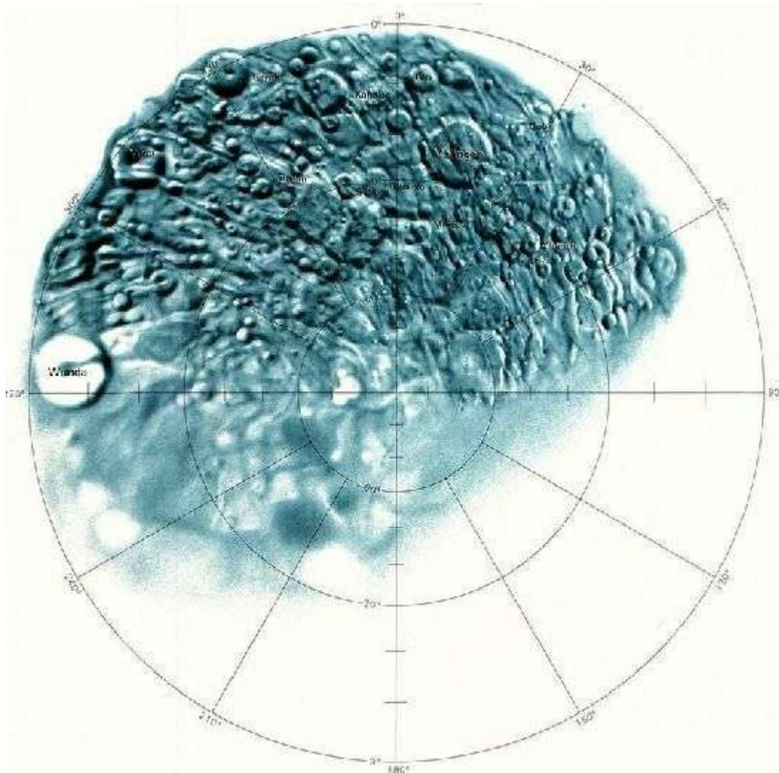
Proyección del polo sur de Umbriel, una de las lunas de Urano. Mapa en relieve sombreado de USGS.
