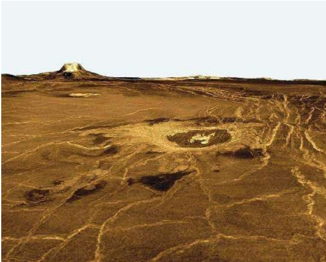
Vistas de las montañas de Venus tomadas por la sonda Magallanes. Cedida por JPL/NASA.
