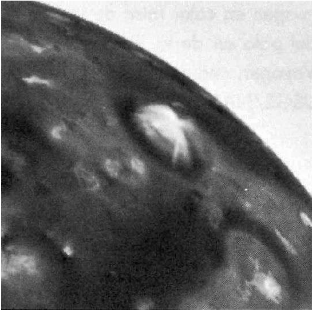
Chorros del volcán Prometheus, en Io, penetrando en la fina atmósfera y cayendo de nuevo al suelo. Datos del Voyager, impresos aquí en negativo para realzar el contraste. Cedita por USGS/NASA.
