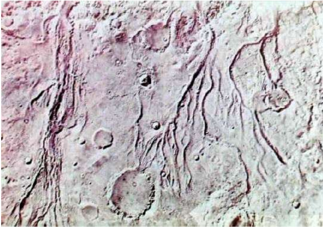
Fotomosaico de una profusa red de valles fluviales. Fotomosaico del Mariner 9, cedido por JPL/NASA.
