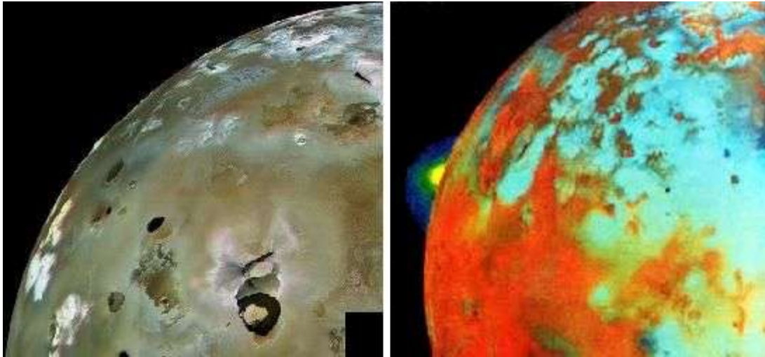
Izquierda: La boca del Loki Patera, en Ío, vista desde arriba (en el centro, abajo). Datos del Voyager, imagen cedida por USGS/NASA. Derecha: El penacho del volcán activo Loki Patera, en la luna Ío, de Júpiter. Datos en color falso del Voyager, cedida por USGS/NASA.
