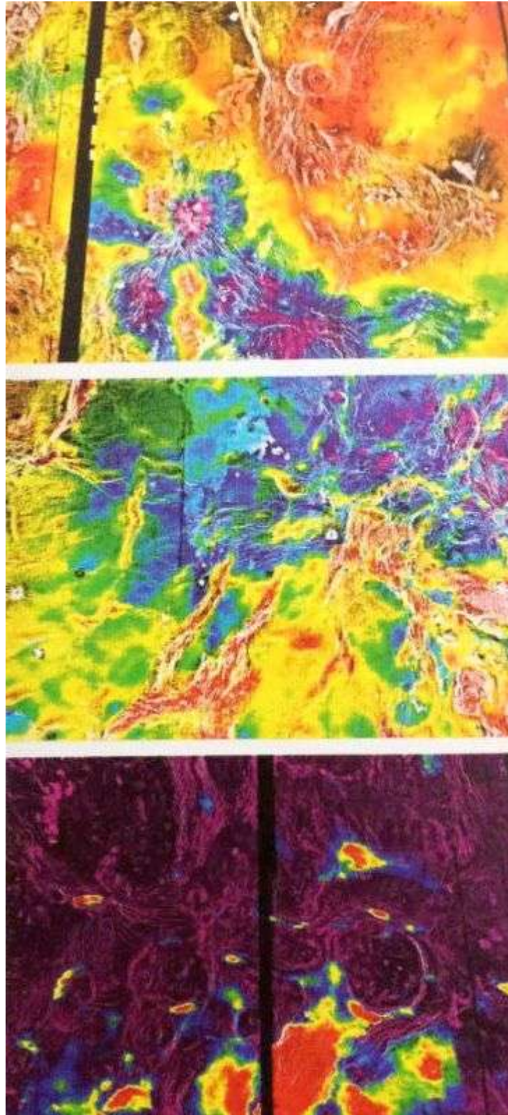
Datos de la sonda espacial Magallanes referentes a la superficie de Venus. Los colores en la imagen central denotan altitud; en la primera
